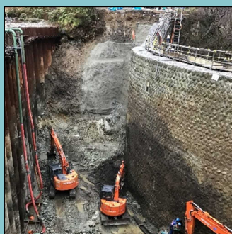
仮締切工 完成
