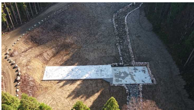
北ノ入川第1号砂防堰堤のH30.11状況 （砂防堰堤の基礎を施工しました。） 写真撮影：（株）種村建設
