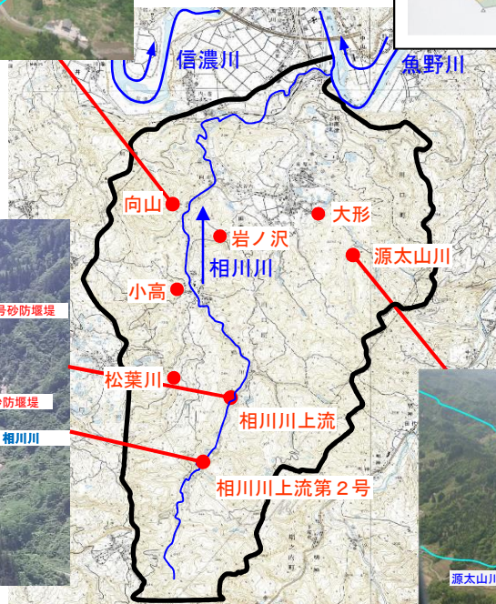
相川川上流砂防堰堤 相川川上流第2号砂防堰堤
