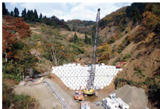
東川砂防えん堤のブロック積施工中のようす 2005.11.18
