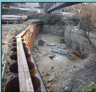
ポンプによる排水
