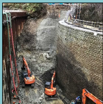
仮締切工 完成
