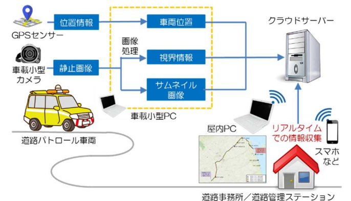
図2 車載カメラ画像収集システムのイメージ
