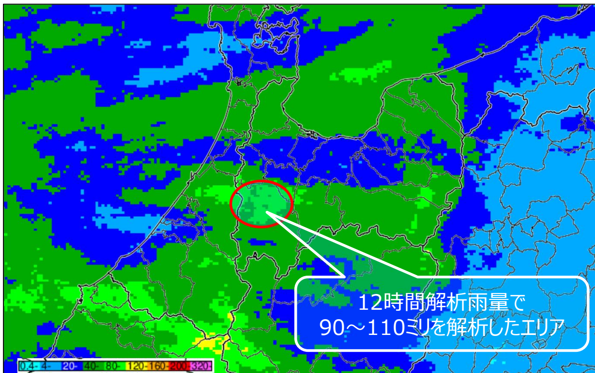
12時間積算解析雨量分布図（7月28日08時00分～28日20時00分）
