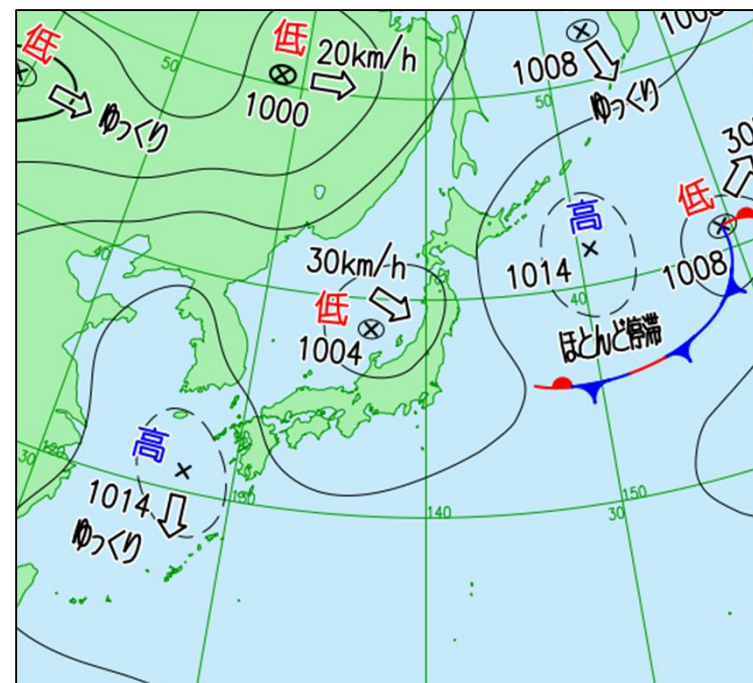
地上天気図（7月28日18時）
