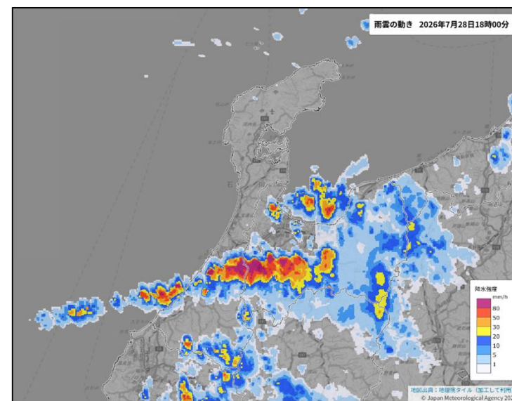
雨雲の動き（7月28日18時）
