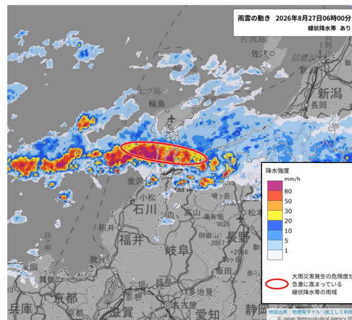
第2図 雨雲の動き（8月27日06時）
