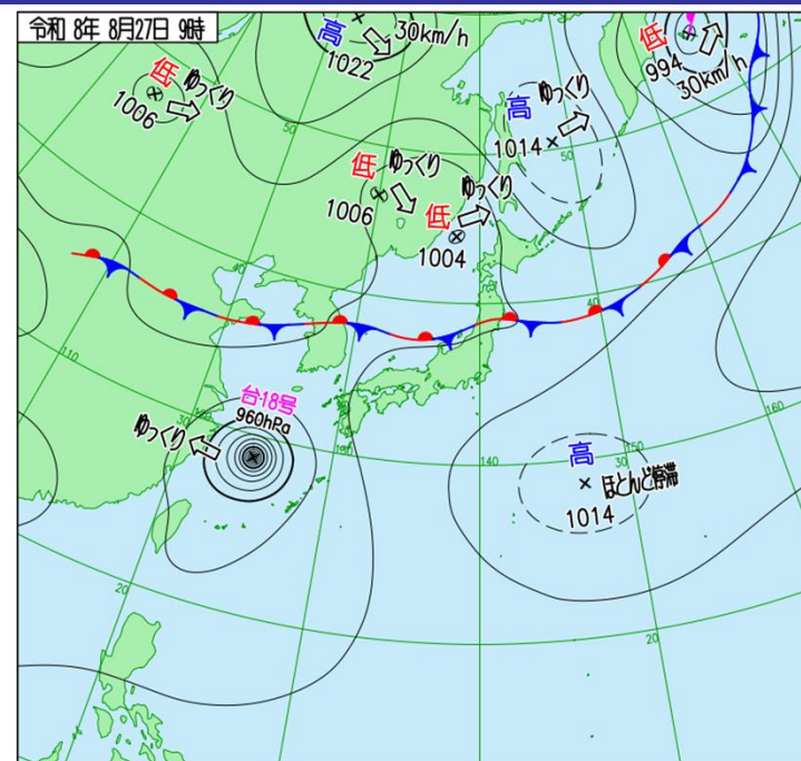
第1図 地上天気図（8月27日09時）
