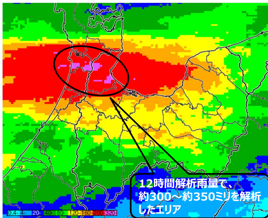
（参考）8月27日09時00分までの12時間積算解析雨量分布図
