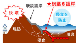
▲ 根継ぎ護岸イメージ図
