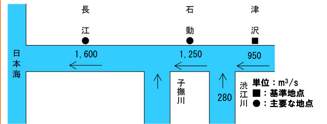
河川整備計画目標流量配分図 (図2-2)
