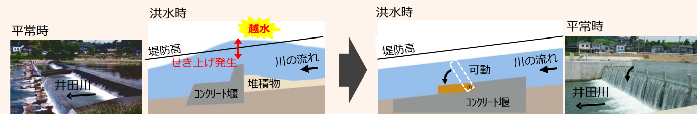
洪水の安全な流下に支障となっていた大坪用水堰の改築（富山市八尾町福島）
