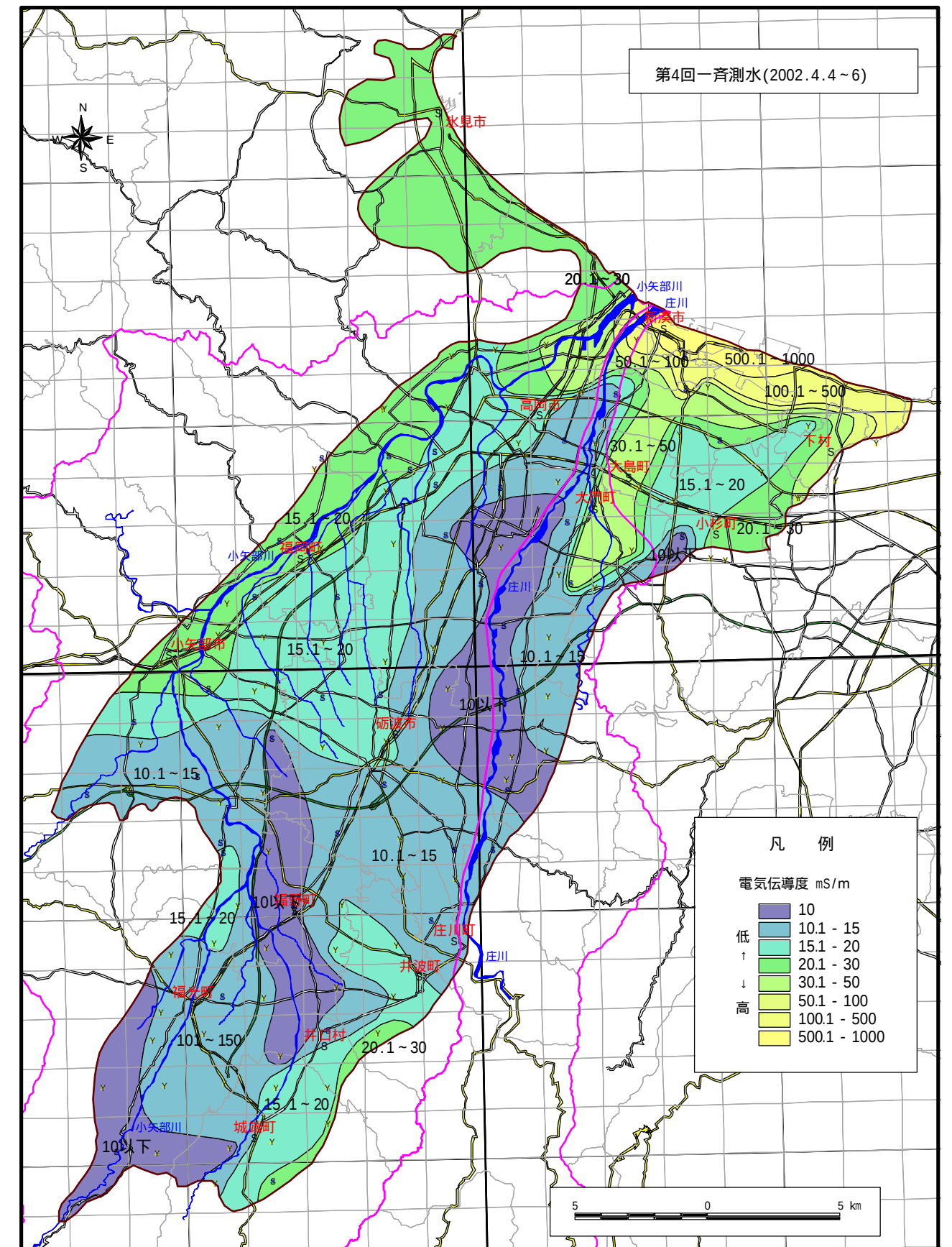
電気伝導度等値線図 (2002年4月)
