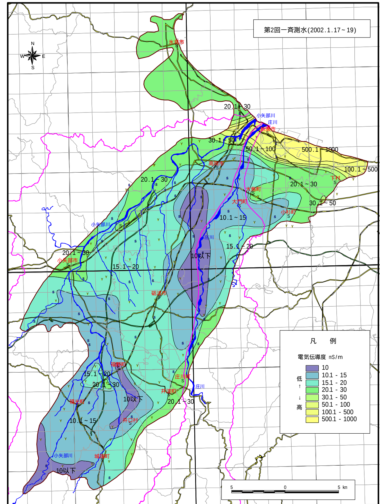
電気伝導度等値線図 (2002年1月)
