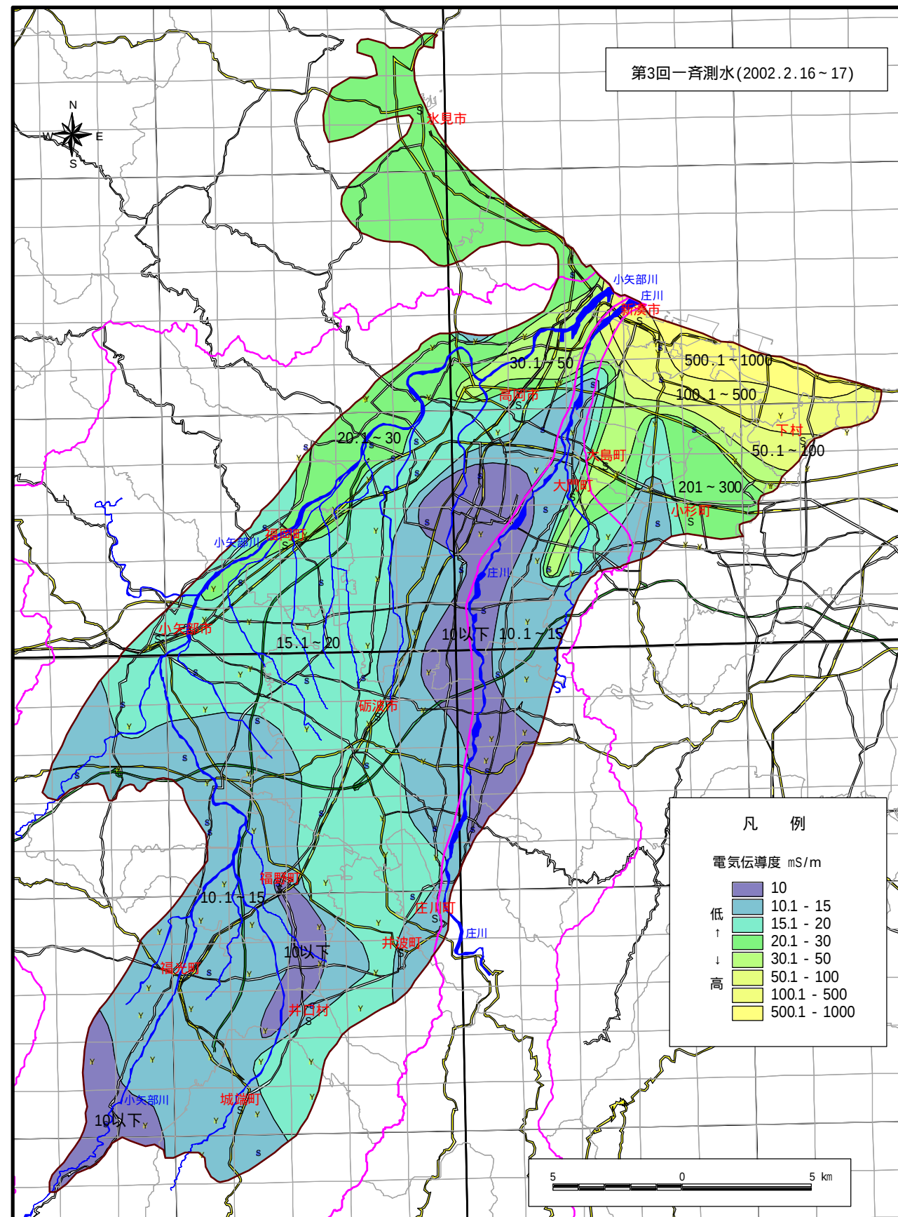
電気伝導度等値線図 (2002年2月)
