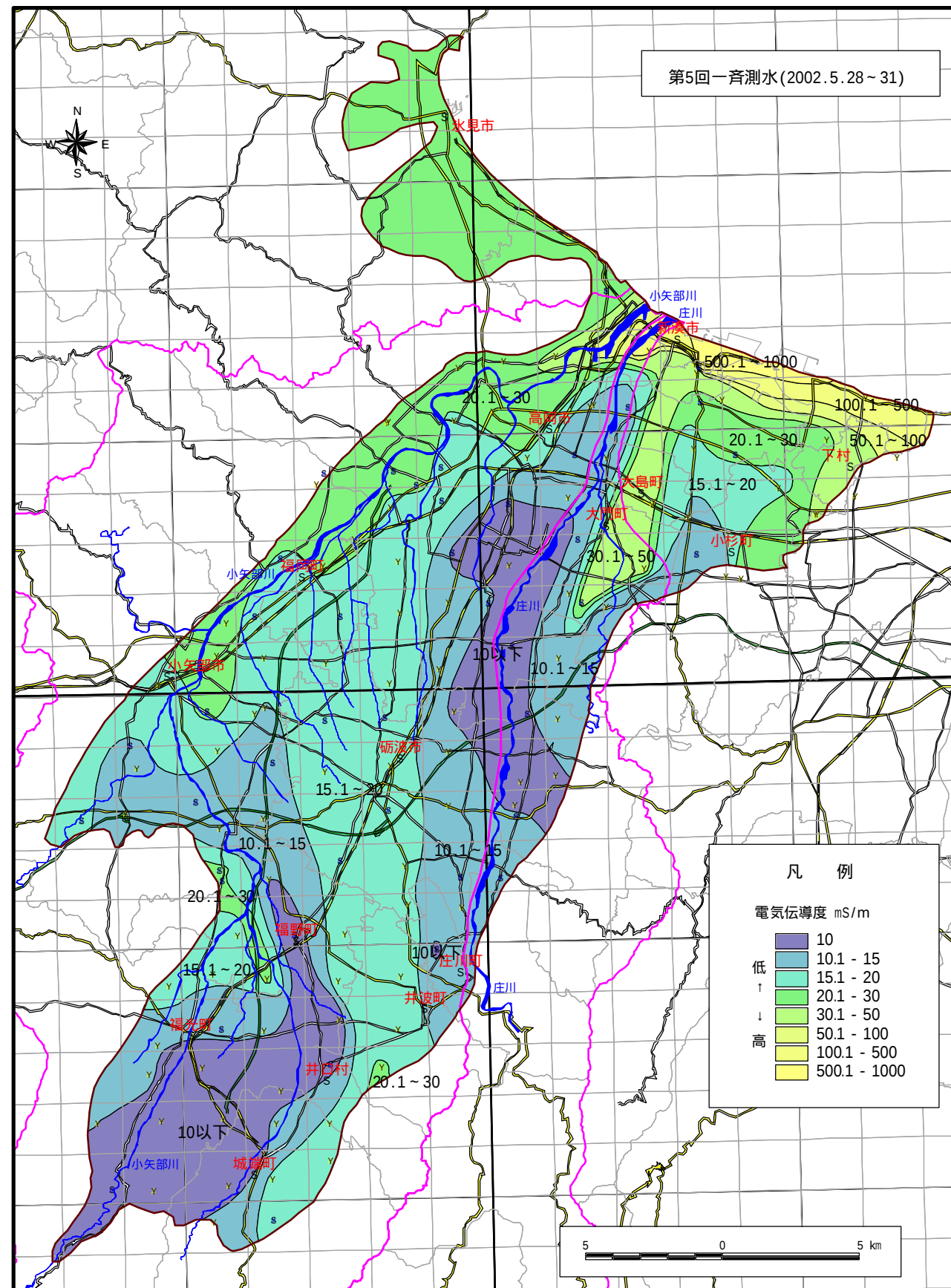
電気伝導度等値線図(2002年5月)
