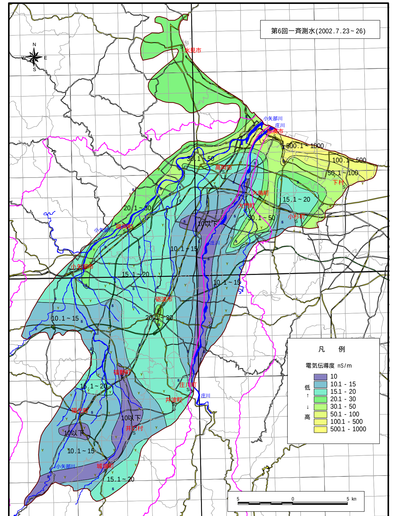
電気伝導度等値線図(2002年7月)
