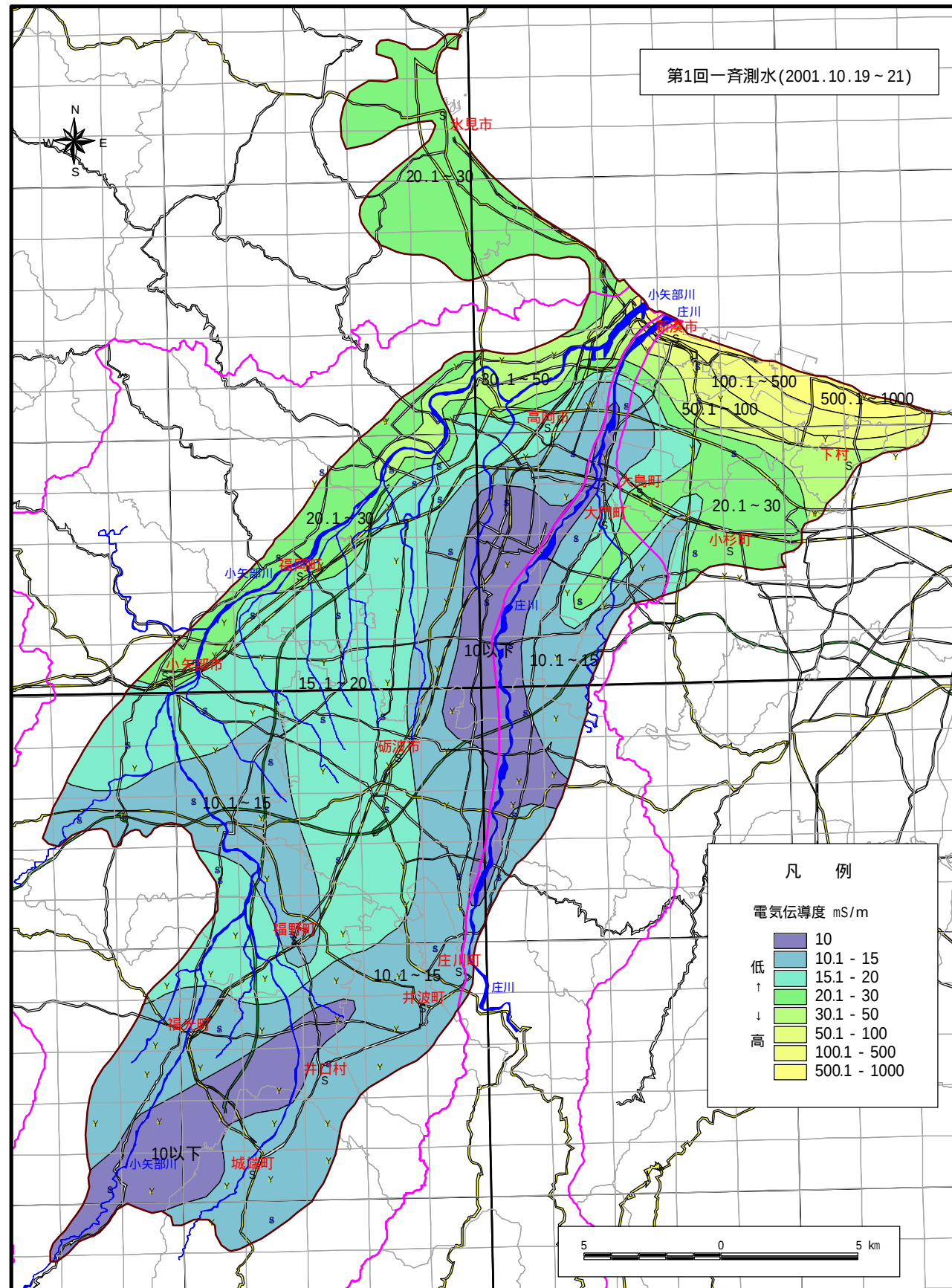
電気伝導度等値線図 (2001年10月)
