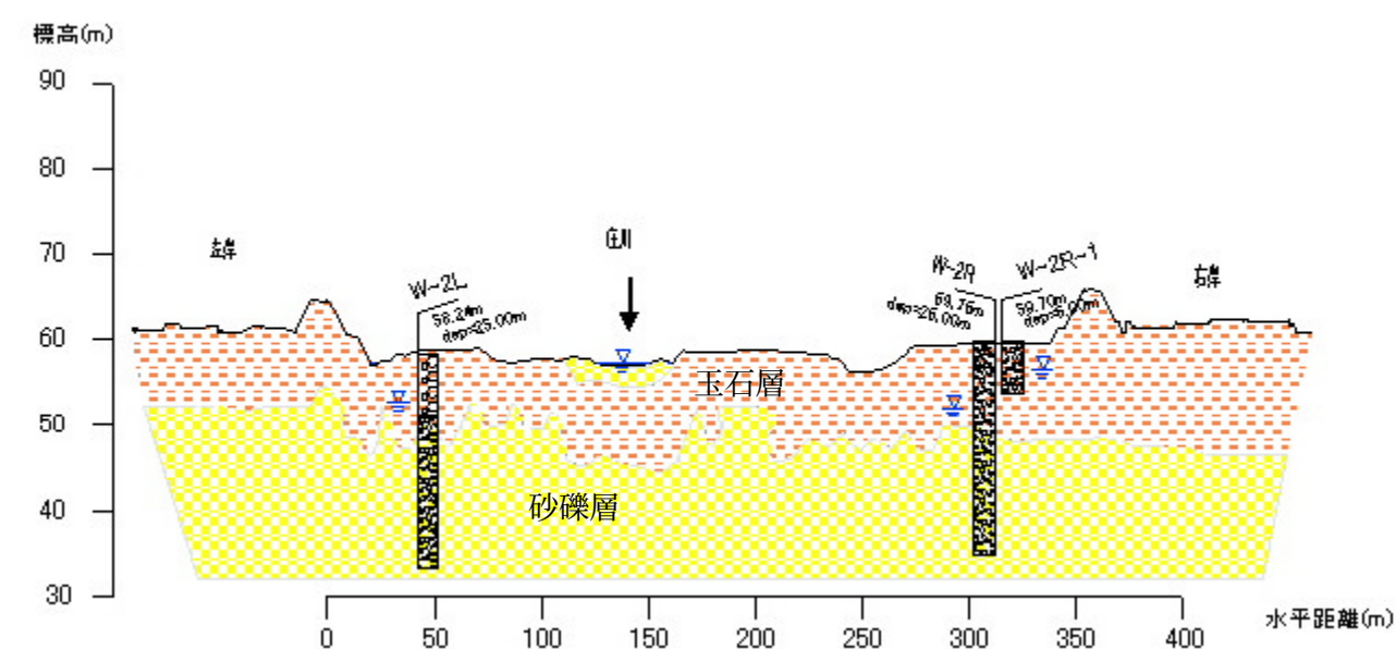
図 3.1-12 本検討による太田橋付近の地質断面図
