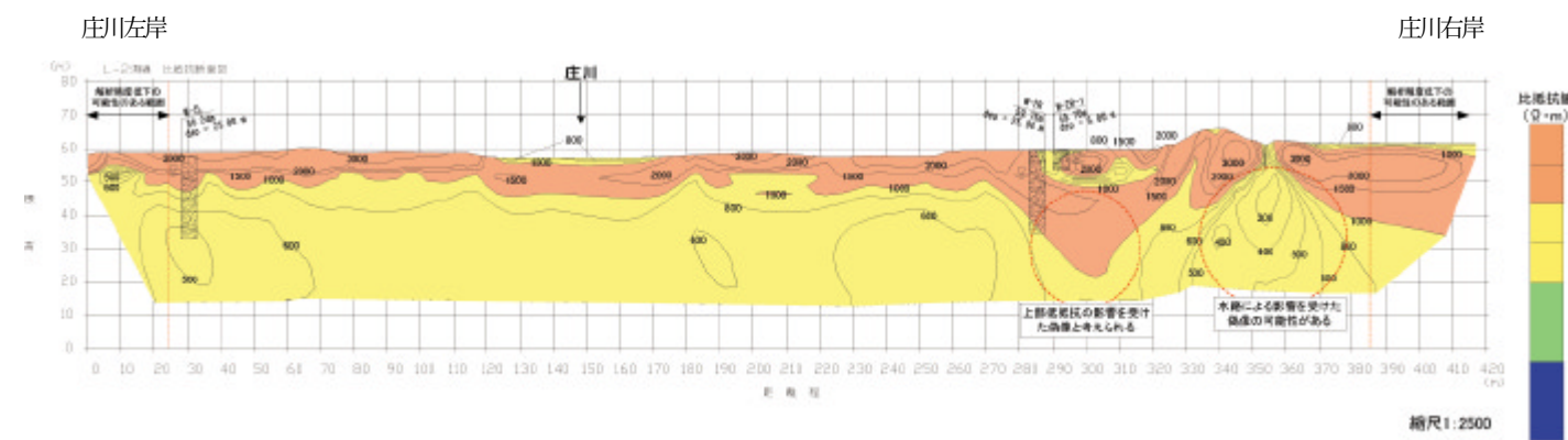
図 3.1-7 太田橋 電気探査結果 (2測線 庄川両岸)
