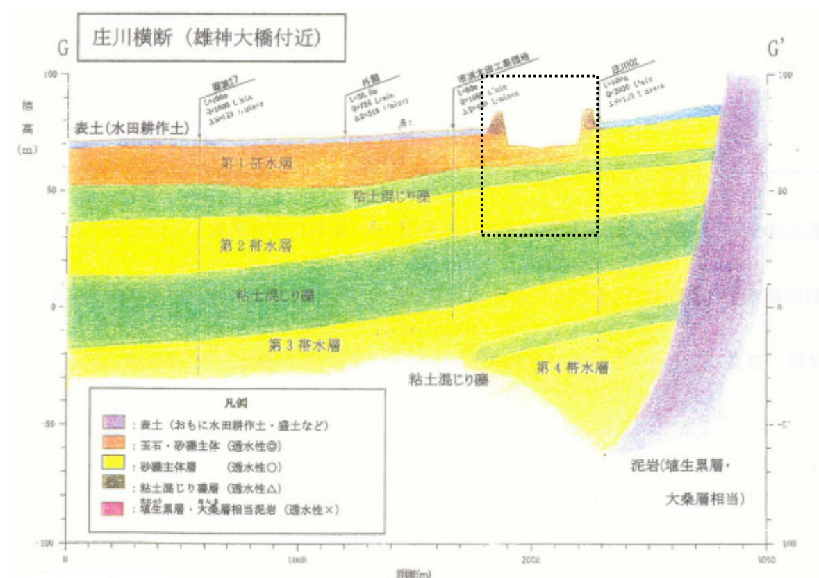
図 3.1-9 雄神大橋付近の水理地質断面図（利賀川工業用水道事業検討会資料、富山県企業局） （参考）（点線は下図の範囲）
