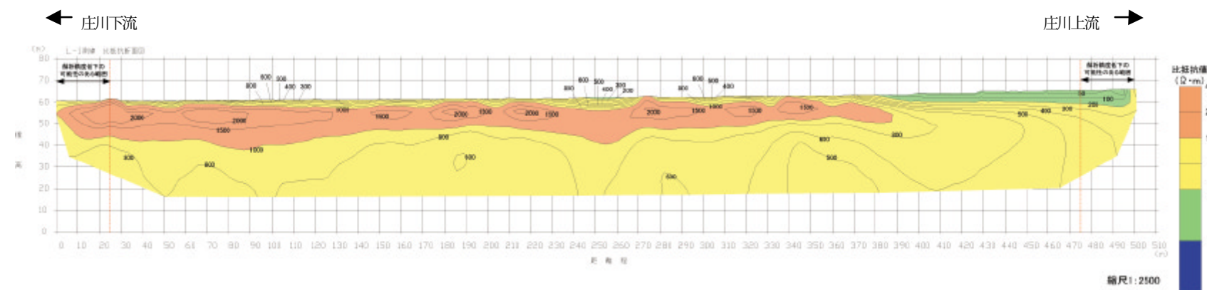
図 3.1-6 太田橋 電気探査結果 (1測線 庄川右岸)
