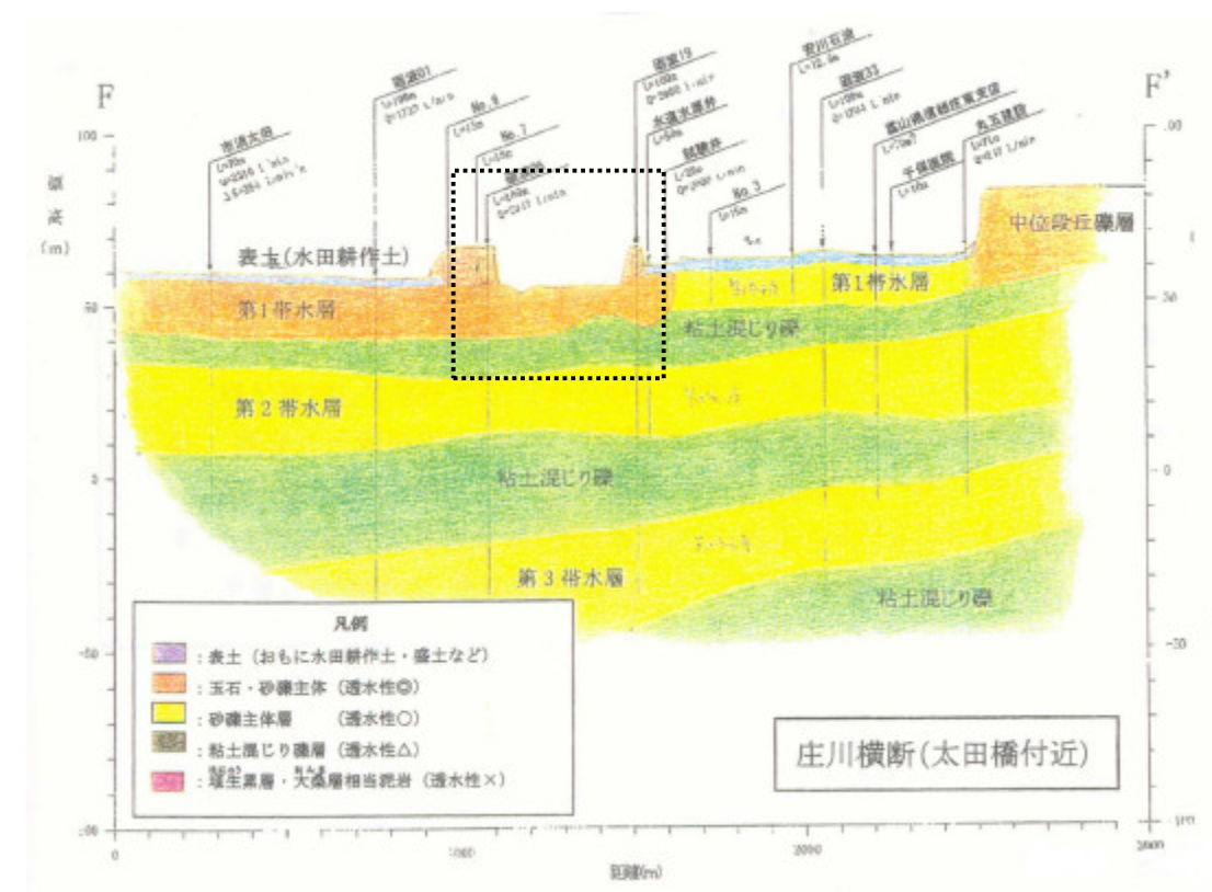
図 3.1-11 太田橋付近の水理地質断面図（利賀川工業用水道事業検討会資料、富山県企業局） （参考）（点線は下図の範囲）
