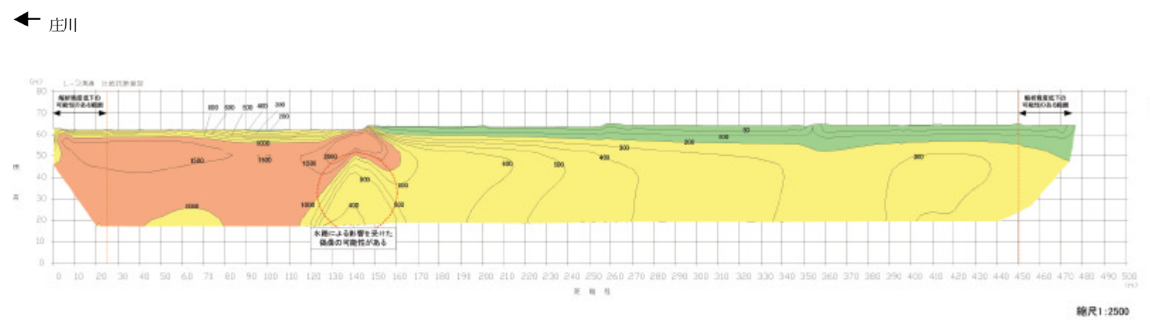
図 3.1-7 太田橋 電気探査結果 (2測線 庄川両岸)
