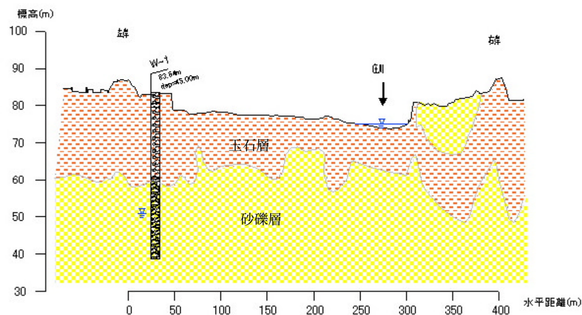
図 3.1-10 本検討による雄神橋付近の地質断面図
