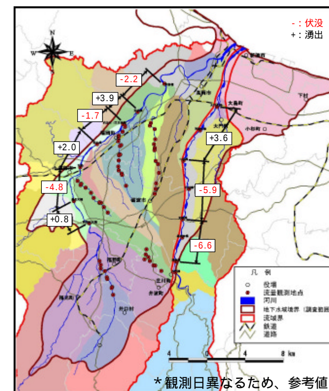
図 2.2-9 同時流量観測結果 (H15.2.4)
