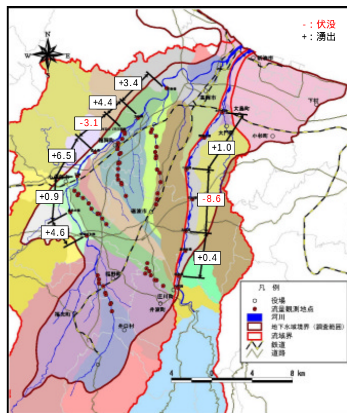
図 2.2-6 同時流量観測結果 (H14.2.8)
