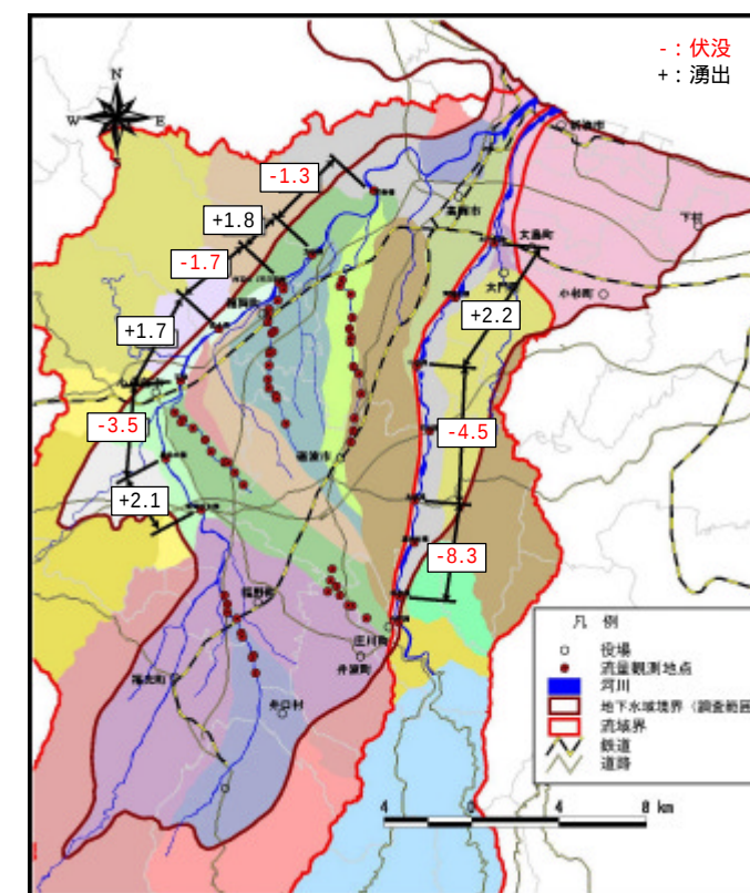
図 2.2-10 同時流量観測結果 (H15.10.30)
