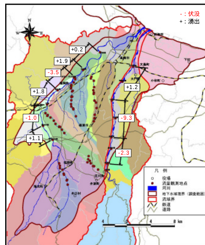
図 2.2-8 同時流量観測結果 (H14.9.25)
