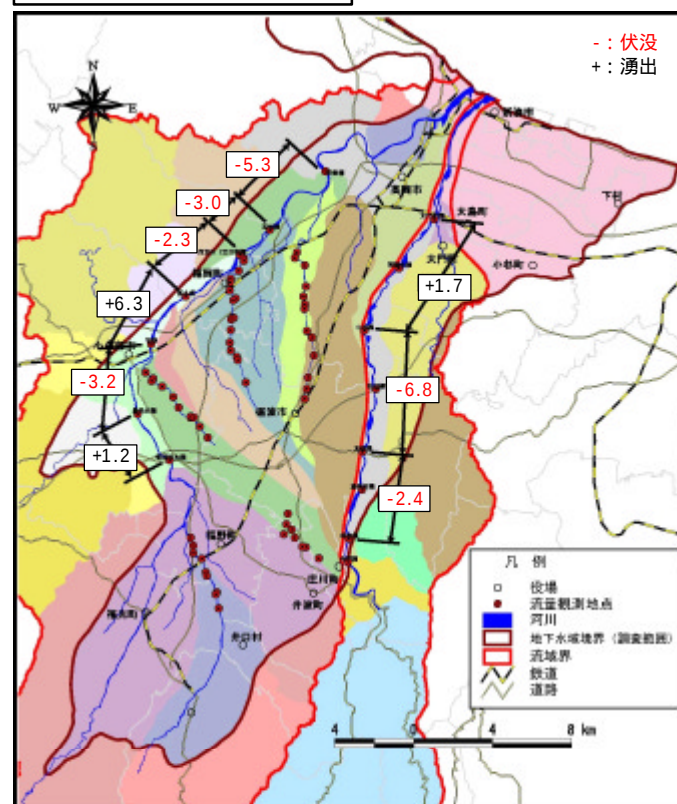
図 2.2-5 同時流量観測結果 (H13.11.1)
