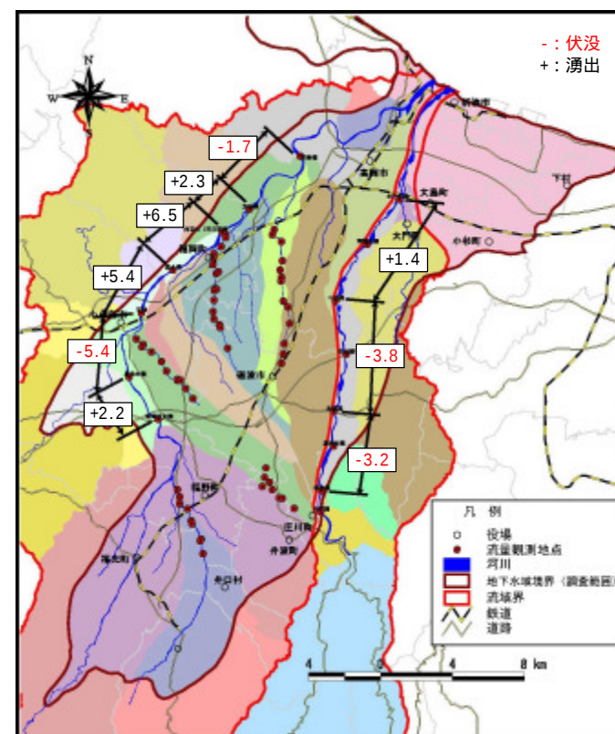
図 2.2-7 同時流量観測結果 (H14.5.30)
