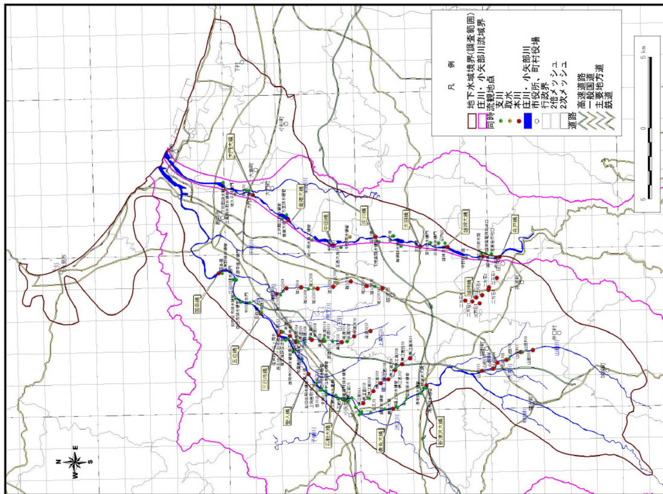
図 2.2-4 同時流量観測地点位置図
