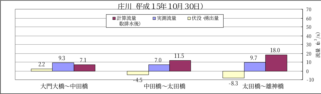
図 2.2-2(2) 庄川の伏没・流出量
