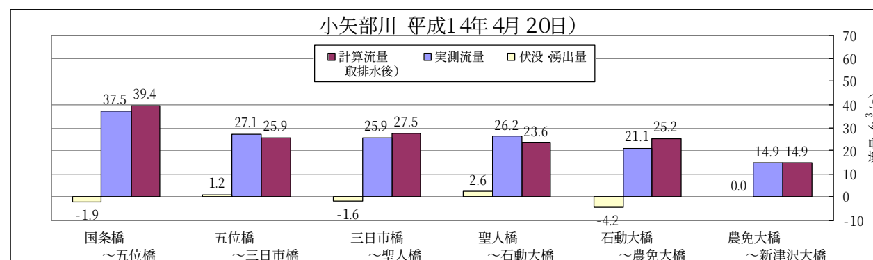
図 2.2-3(1) 小矢部川の伏没・湧出量
