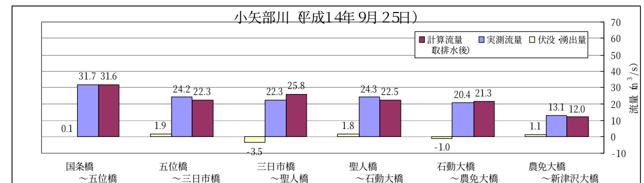
図 2.2-3(1) 小矢部川の伏没・湧出量
