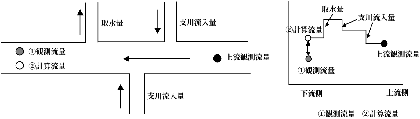
図 2.2-1 伏没・湧出量の算定模式図
