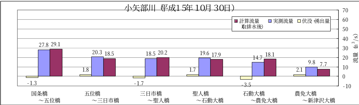
図 2.2-3(2) 小矢部川の伏没・湧出量
