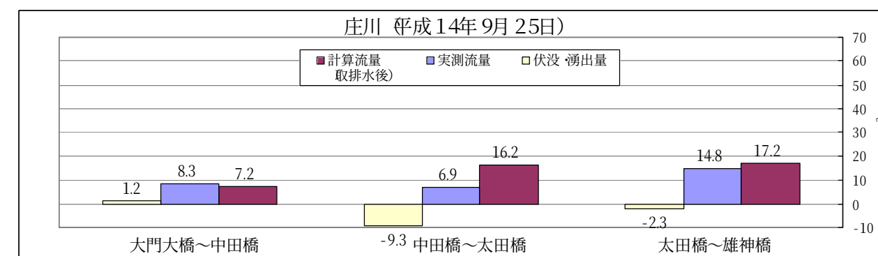
図 2.2-2(1) 庄川の伏没・流出量
