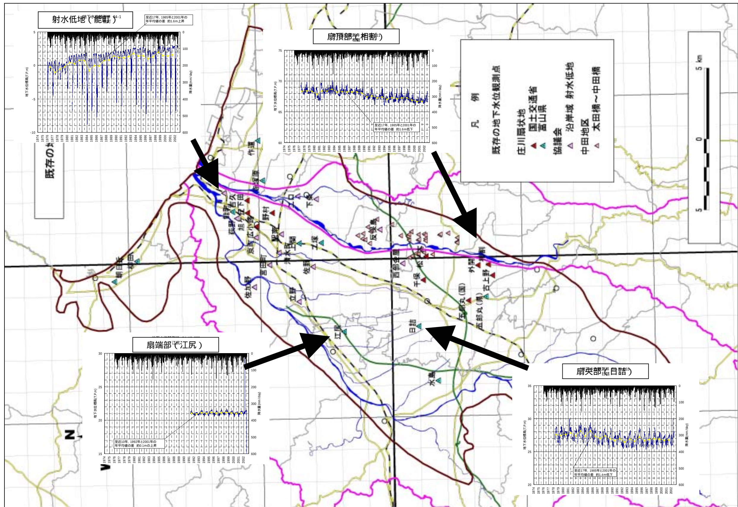
図 2-5-2 砺波平野の地下水観測態勢と地下水位変動
