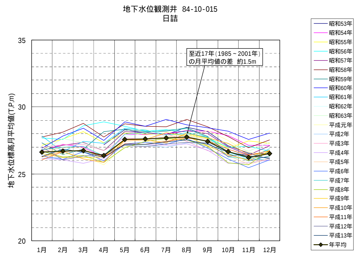
図 2-5-3 (2) 地下水位の経年変化(上)月変化(下) [ 扇中部 ]
