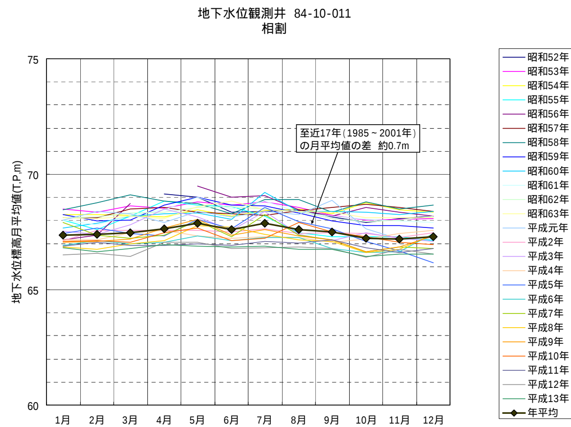
図 2-5-3 (1) 地下水位の経年変化(上)月変化(下) [ 扇頂部 ]
