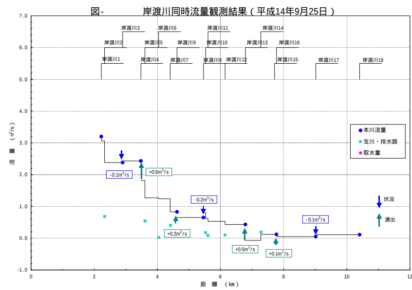
図 2-2-9（6） 同時流量観測結果（水収支縦断図）
