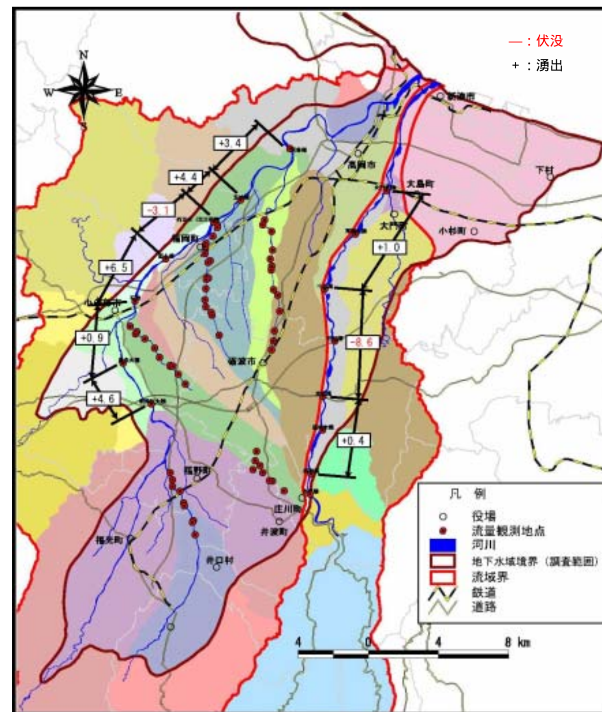
図 2-2-6 同時流量観測結果 (H14.2.8)
