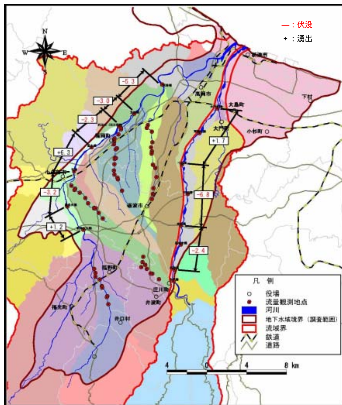
図 2-2-5 同時流量観測結果 (H13.11.1)
