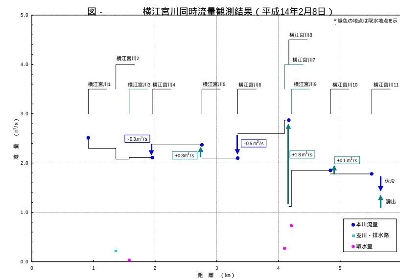
図 2-2-9 (1) 同時流量観測結果（水収支縦断図）
