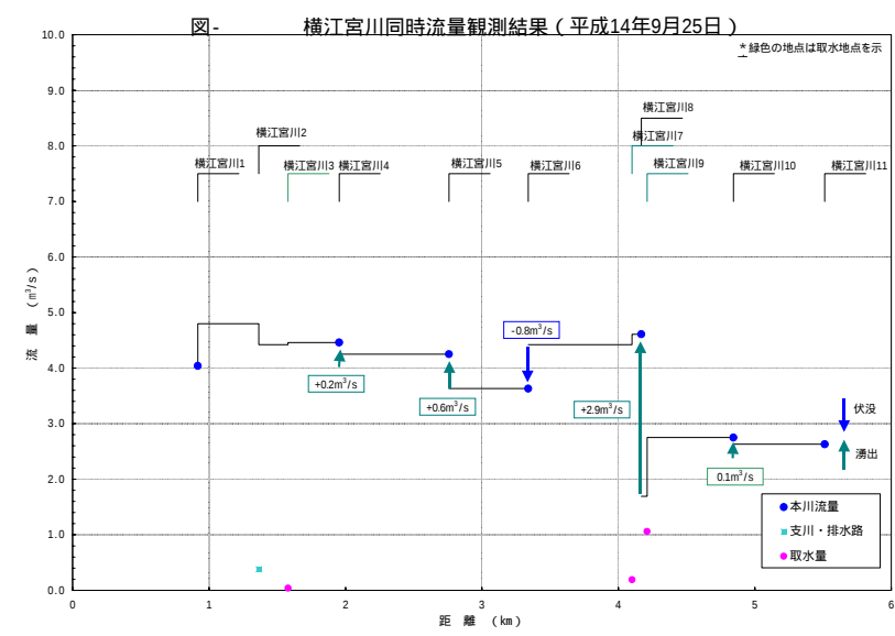
図 2-2-9（5） 同時流量観測結果（水収支縦断図）
