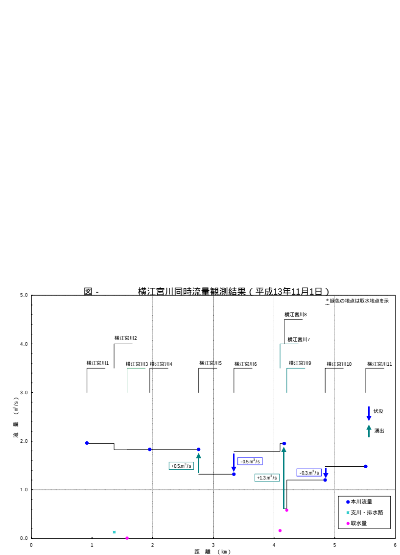
横江宮川同時流量観測結果水収支縦断図
