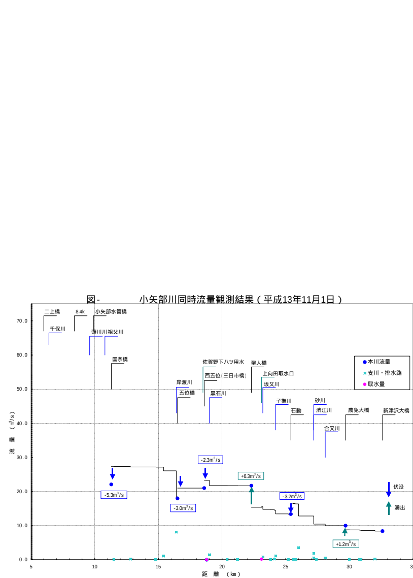
小矢部川同時流量観測結果水収支縦断図
