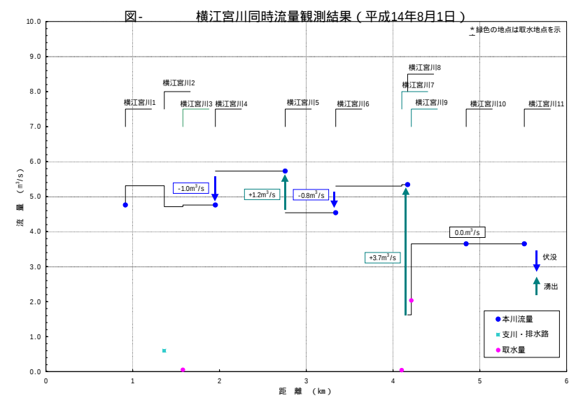
横江宮川同時流量観測結果水収支縦断図
