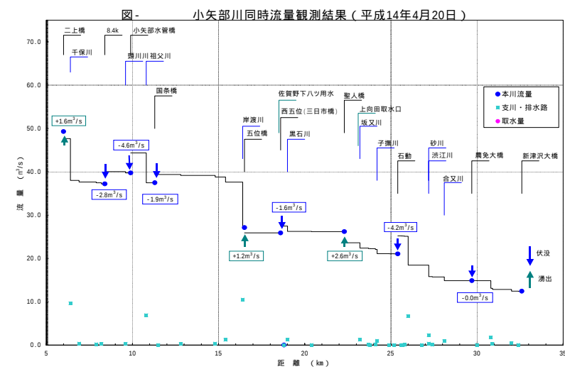
小矢部川同時流量観測結果水収支縦断面図
