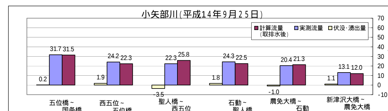
図 2-2-3 小矢部川の伏没・湧出量
