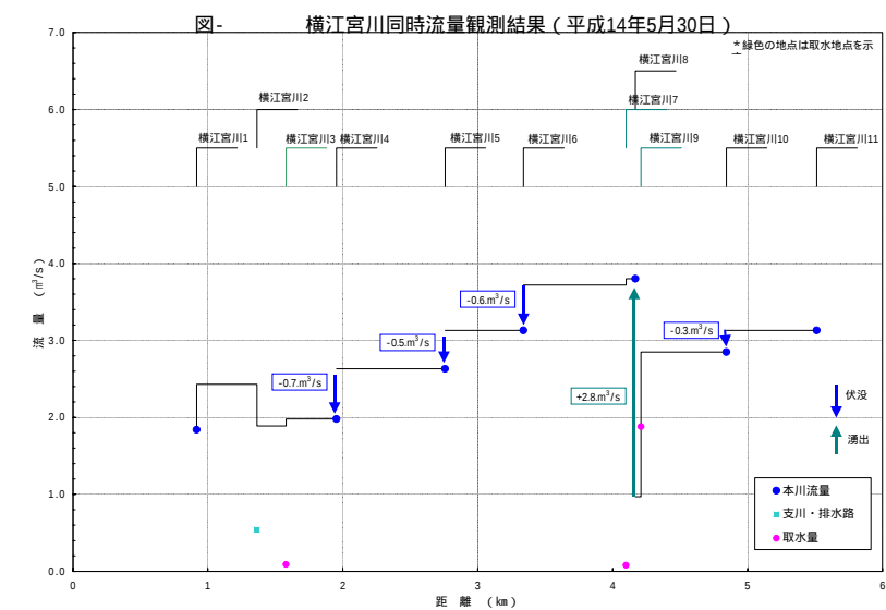
図 2-2-9 (3) 同時流量観測結果（水収支縦断面図）
