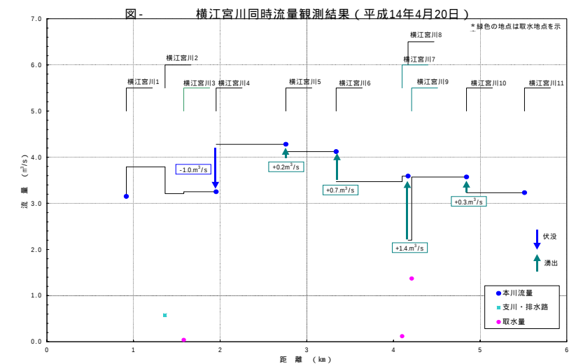
横江宮川同時流量観測結果水収支縦断面図
