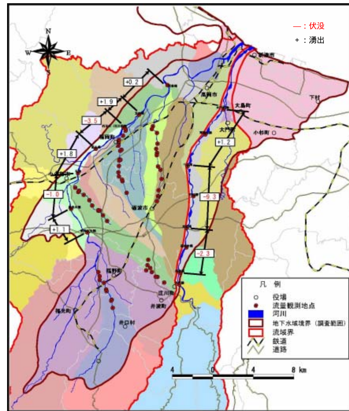
図 2-2-8 同時流量観測結果 (H13.9.25)
