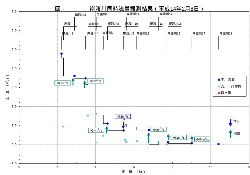
図 2-2-9（2） 同時流量観測結果（水収支縦断図）
