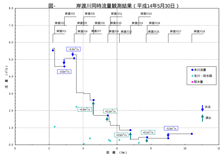
図 2-2-9 (4) 同時流量観測結果（水収支縦断図）
