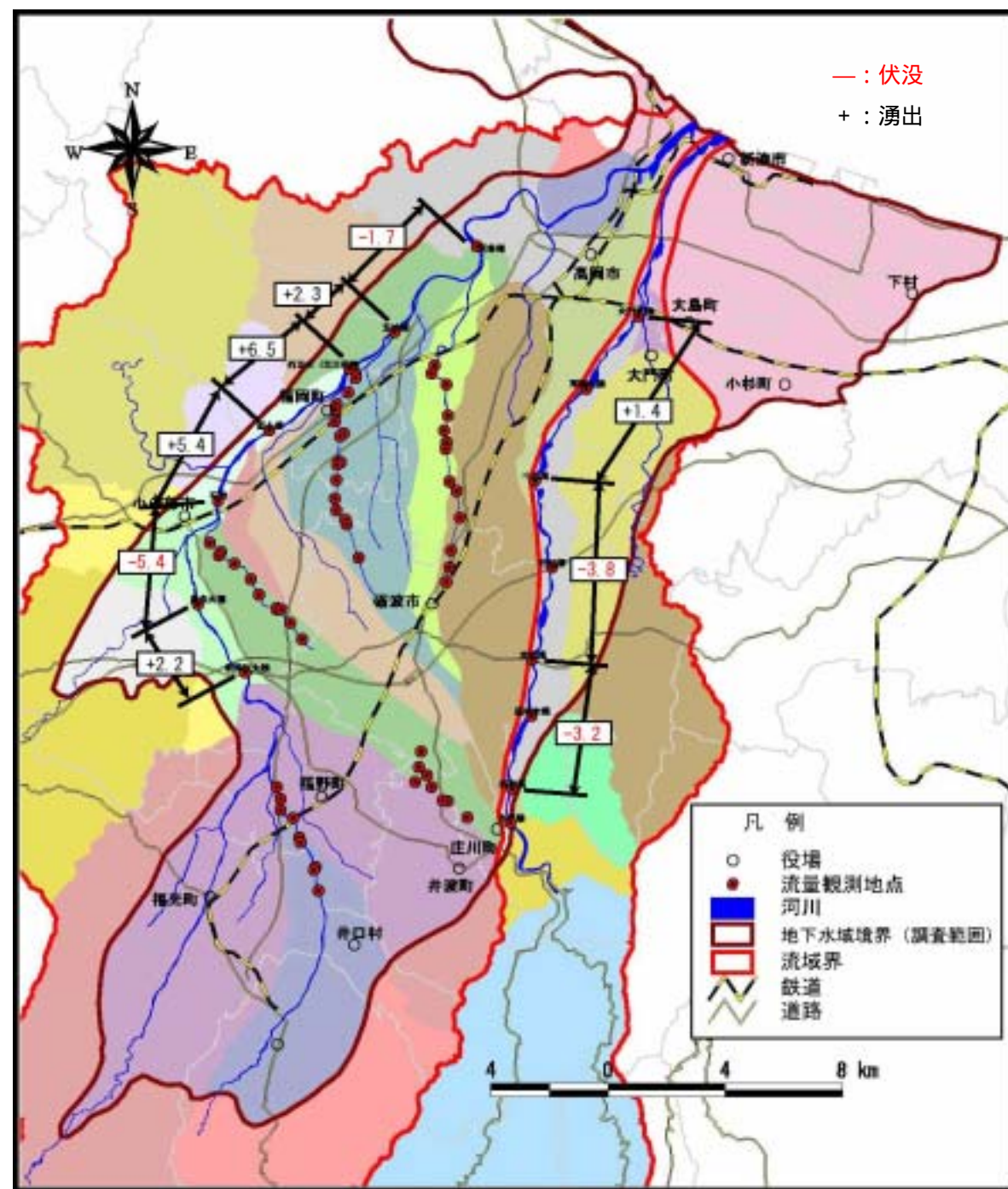
図 2-2-7 同時流量観測結果 (H14.5.30)
