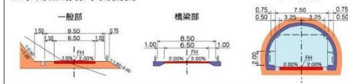
工事用道路標準断面図
