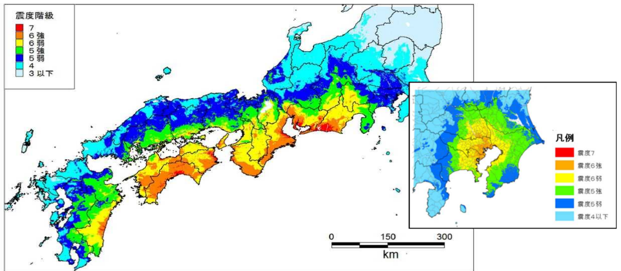
図 21 南海トラフ巨大地震及び首都直下地震の震度分布
