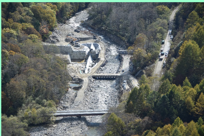
環境に配慮した砂防堰堤を施工中 (真川上流第1号砂防堰堤)
