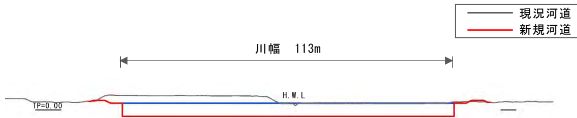
図 2.3.2 代表断面図（1.8k 付近）
