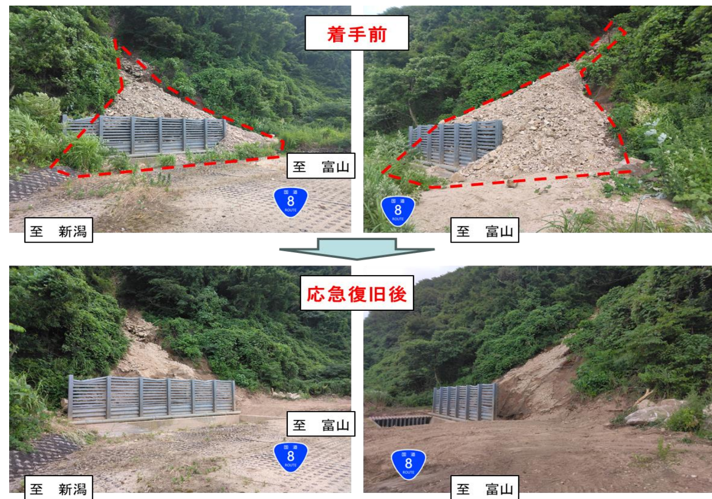
勝山8号洞門上 進捗写真
