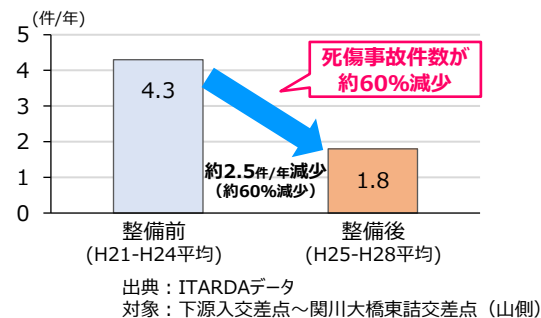
【山側3車線化H24開通区間の事故削減効果】
