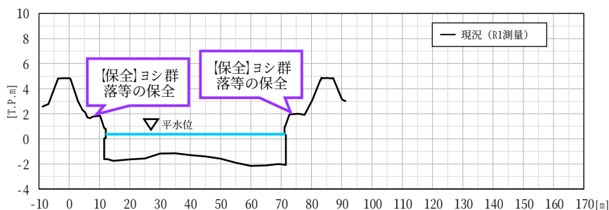
図 5-7 関川における河道掘削横断イメージ (2/2)
