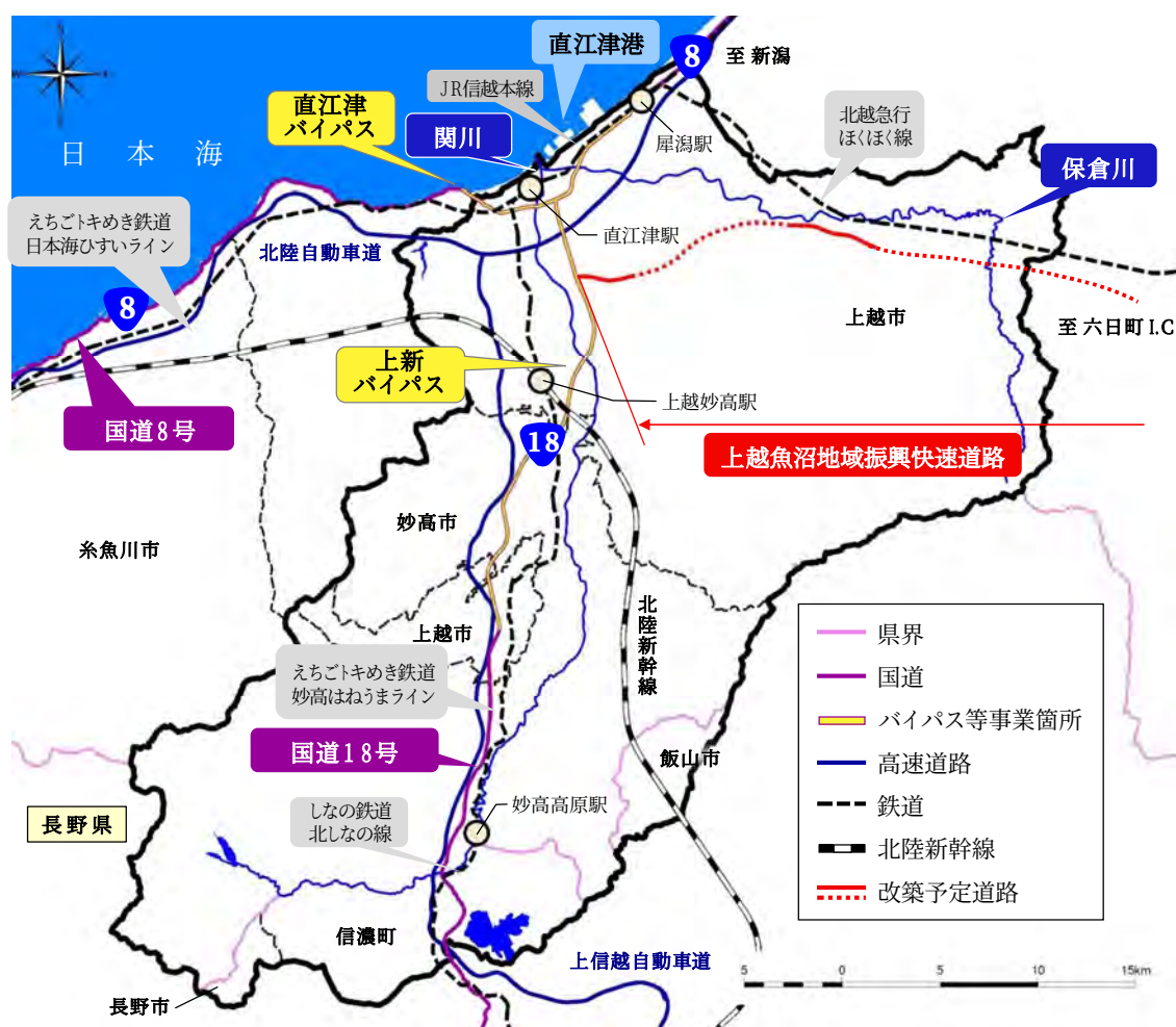
図 2-13 交通体系図
