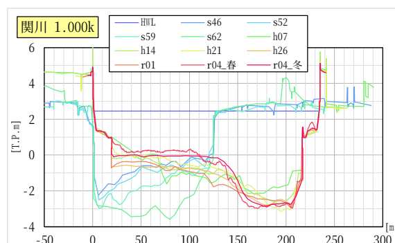
図 5-9 河川定期横断測量
