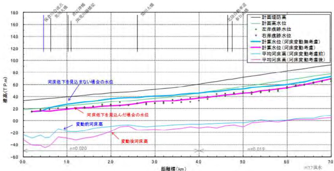
図 5-10 H7.7 洪水 水位縦断図（高田地点 Q=2,600 \text{ m}^3/\text{s} ）
