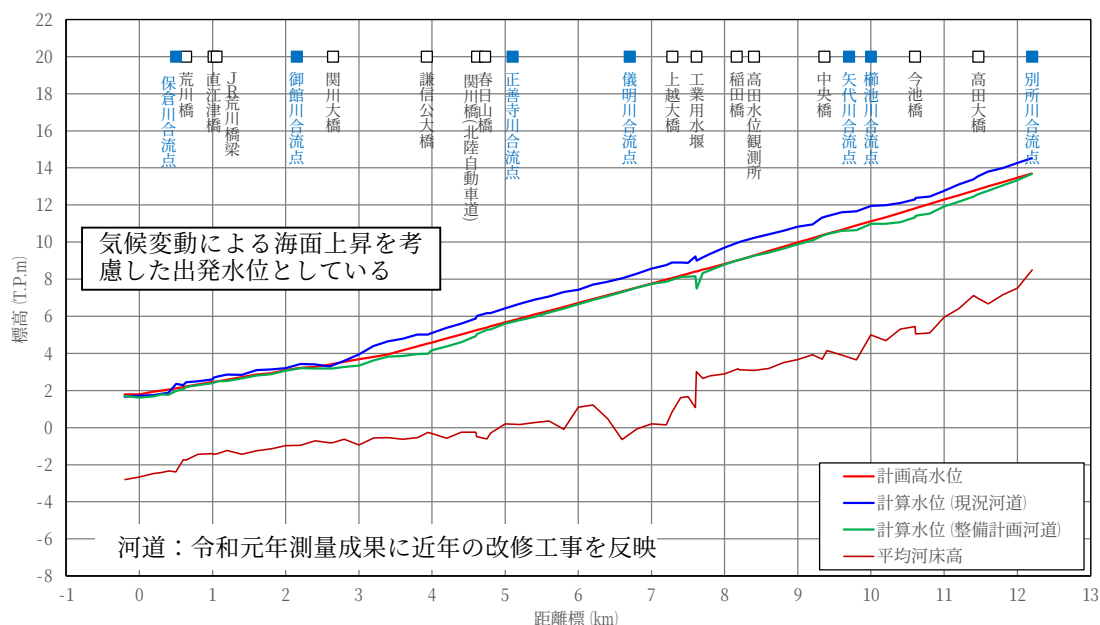
図 3-2 関川の縦断水位（整備計画流量流下時）
