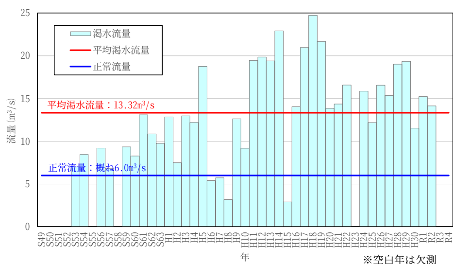
図 3-15 高田地点における渇水流量の経年変化
