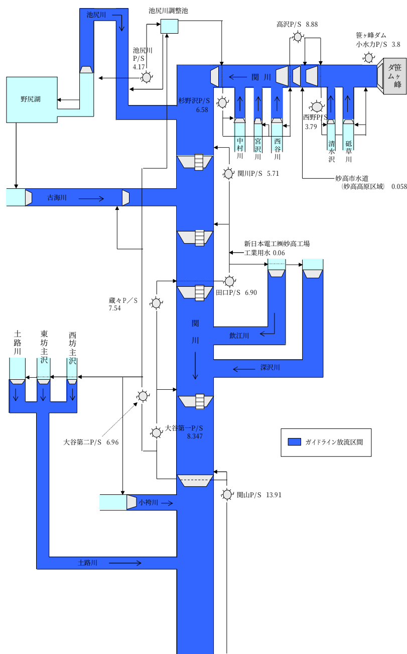
図 5-6 関川水利模式図(1/2) (令和5年(2023年)8月現在)
