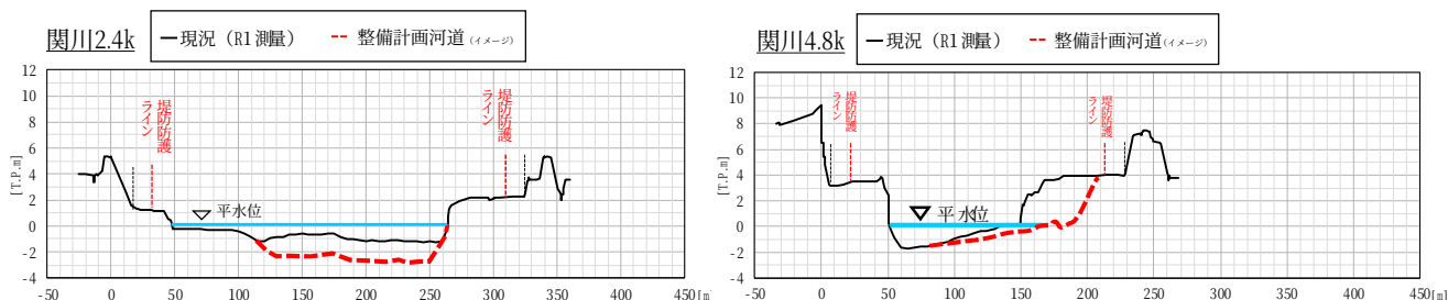
※掘削箇所や掘削断面（または、掘削形状）については、今後の詳細設計を経て最終的な形状を決定 図 5-5 主要な地点の計画横断形状イメージ図
