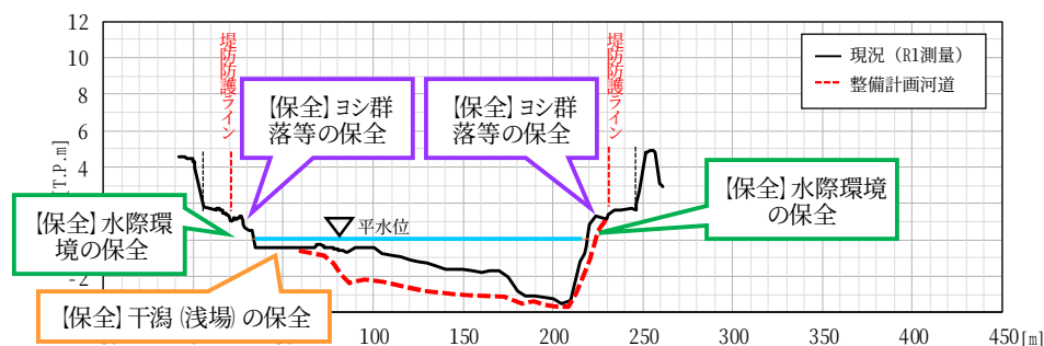
図 5-7 関川における河道掘削横断イメージ（1/2）
