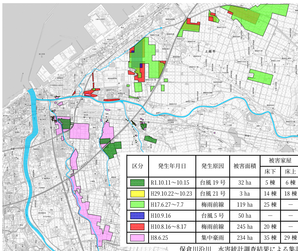
図 3-1 平成 8 年（1996 年）以降の浸水被害実績
