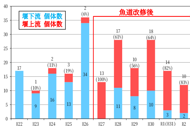
図 3-24 上越工業用水道取水堰堤上下流のサケ確認数の経年変化
