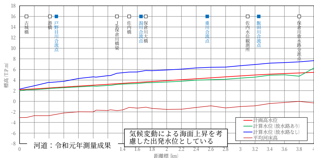
図 3-3 保倉川の縦断水位（整備計画流量流下時）
