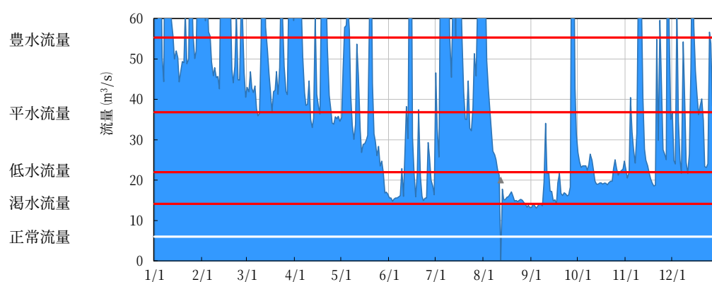
図 3-16 令和 2 年（2020 年）の流況（高田地点）
