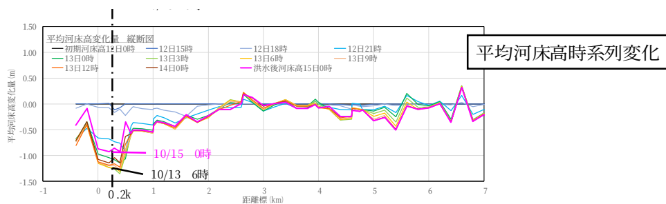
図3-7 河床変動シミュレーション結果(令和元年(2019年)10月洪水)
