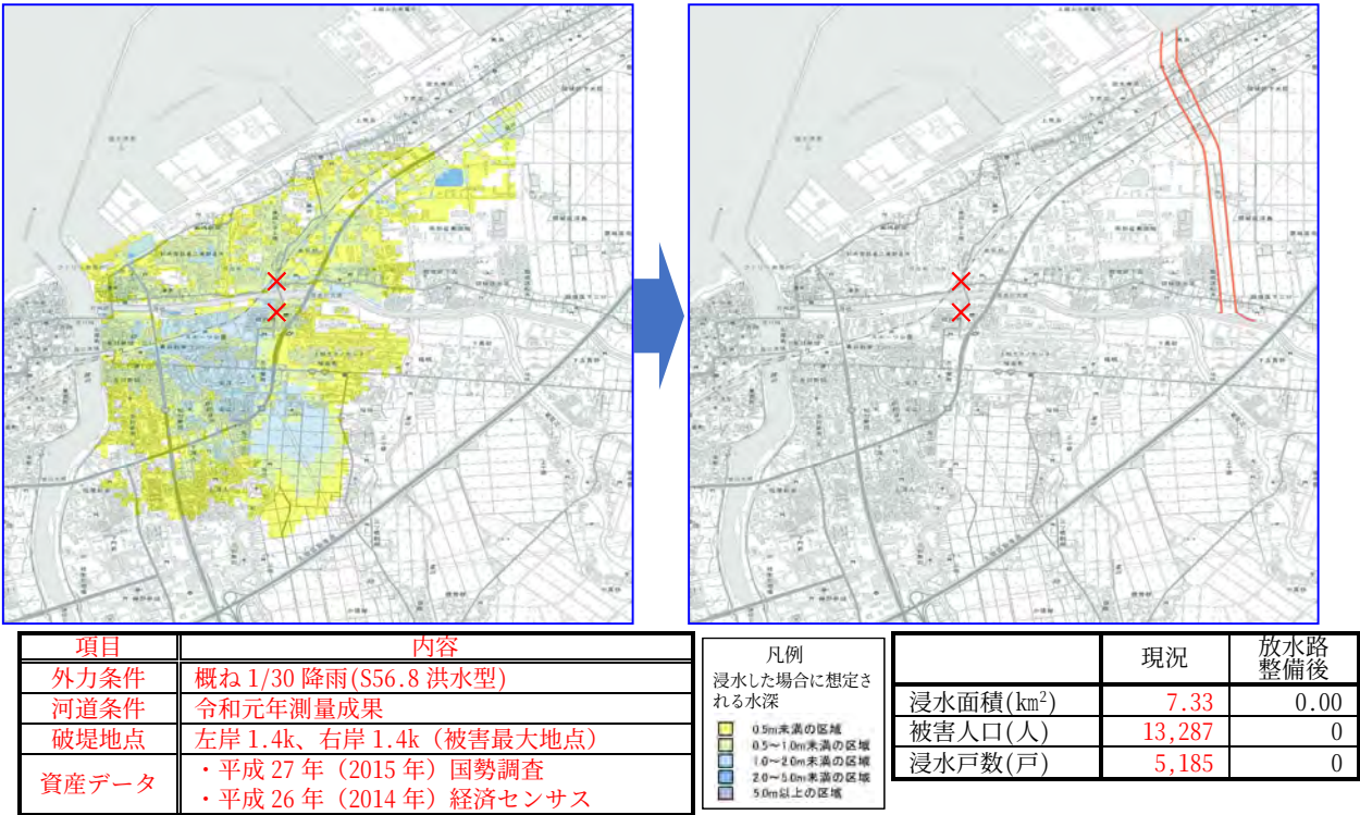
図 5-4 保倉川洪水氾濫シミュレーション結果 (変更整備計画)
