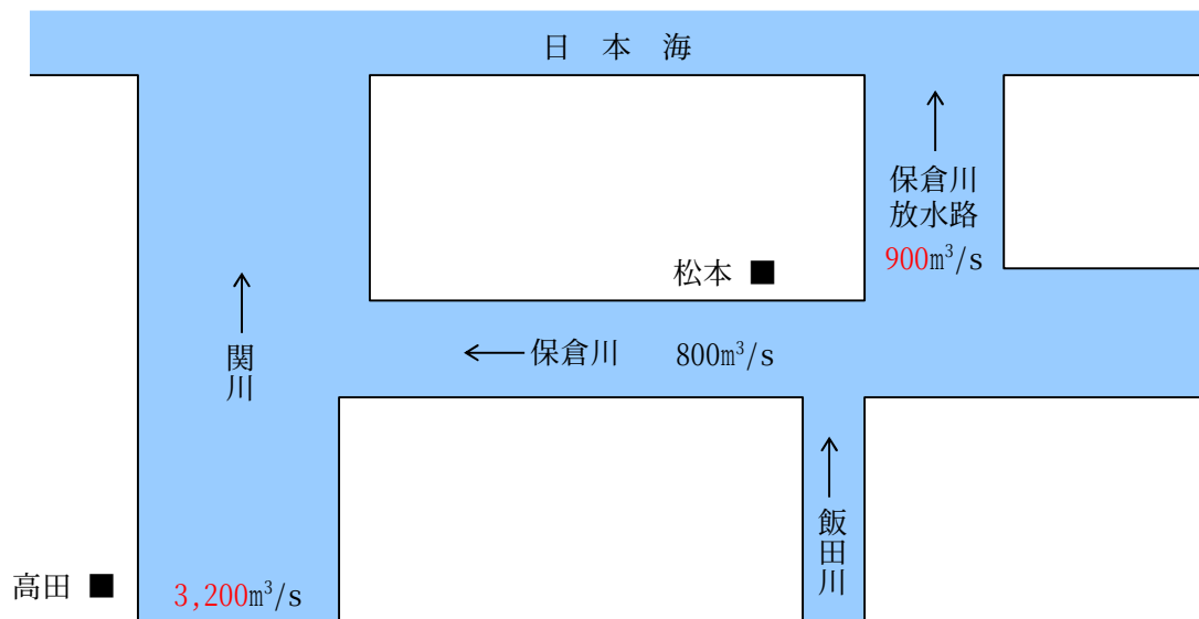
図 4-1 基準地点における河道配分流量
