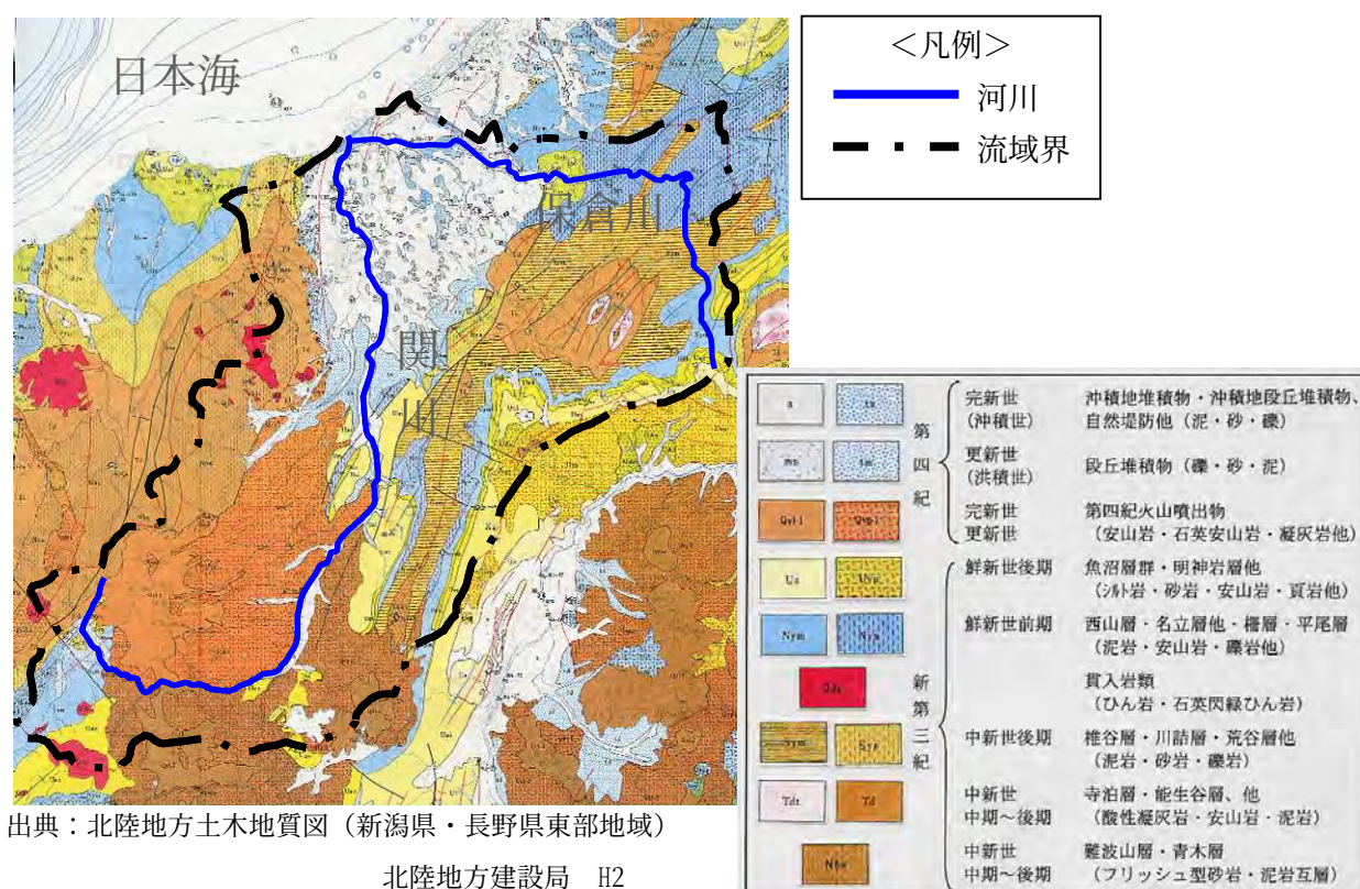
図 2-2 関川流域地質図
