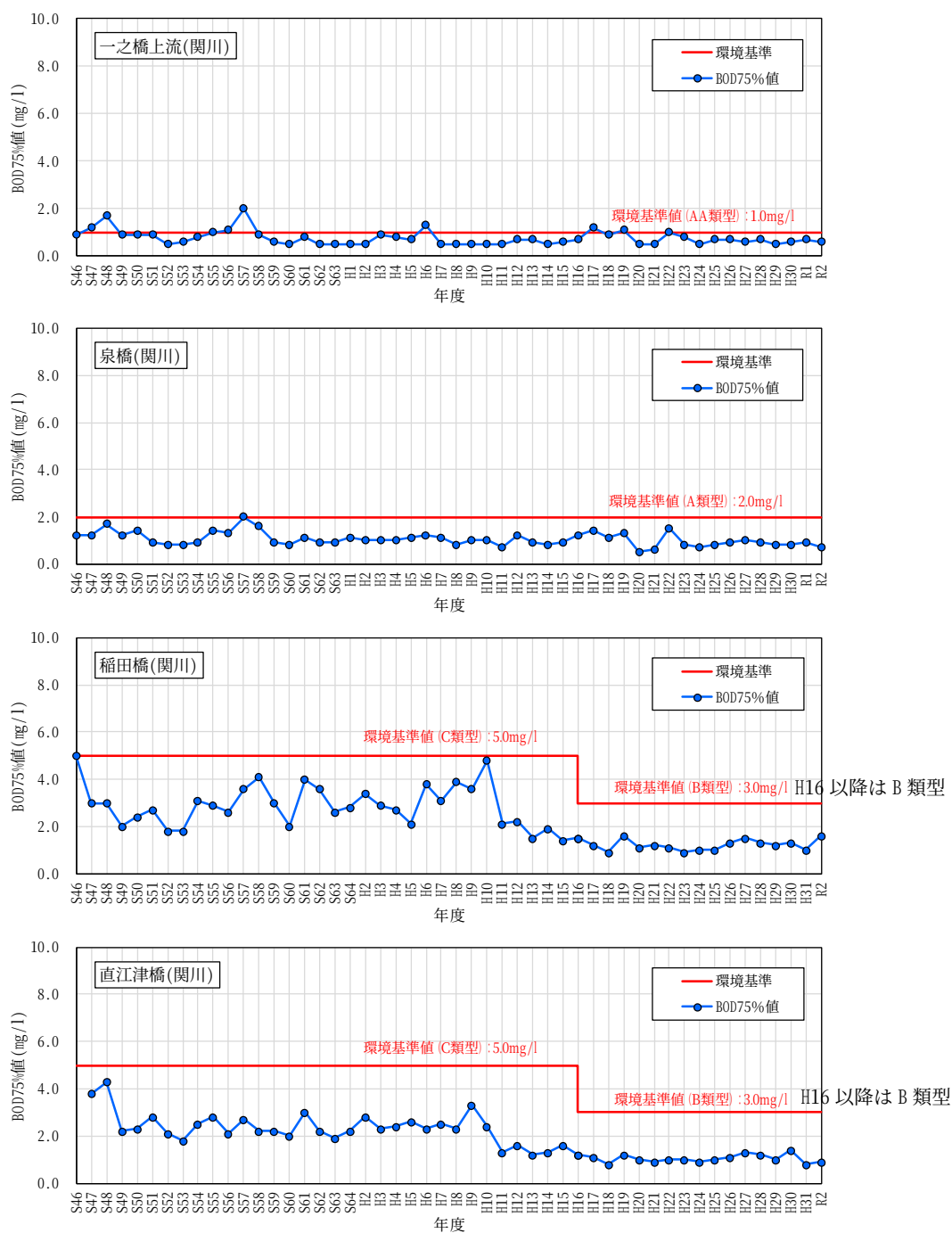
図 3-21 関川の各地点における水質（BOD75%値）の経年変化
