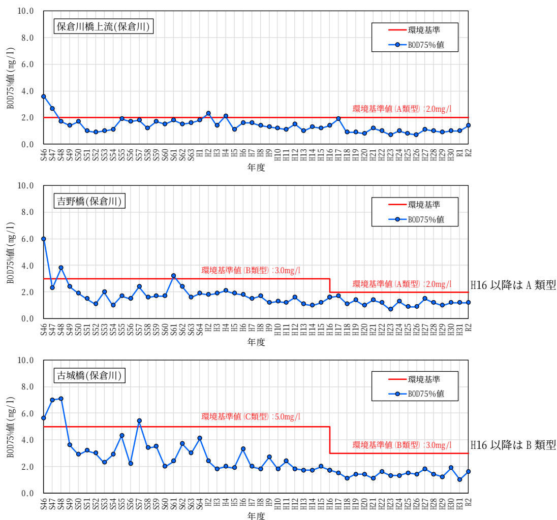
図 3-22 保倉川の各地点における水質（BOD75%値）の経年変化
