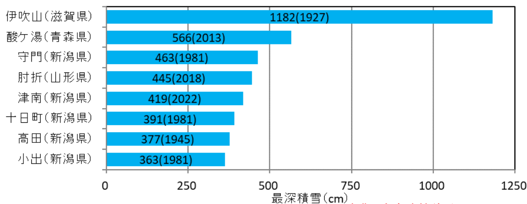
図 2-4 積雪の最深記録 (統計開始から令和4年(2022年)まで)
