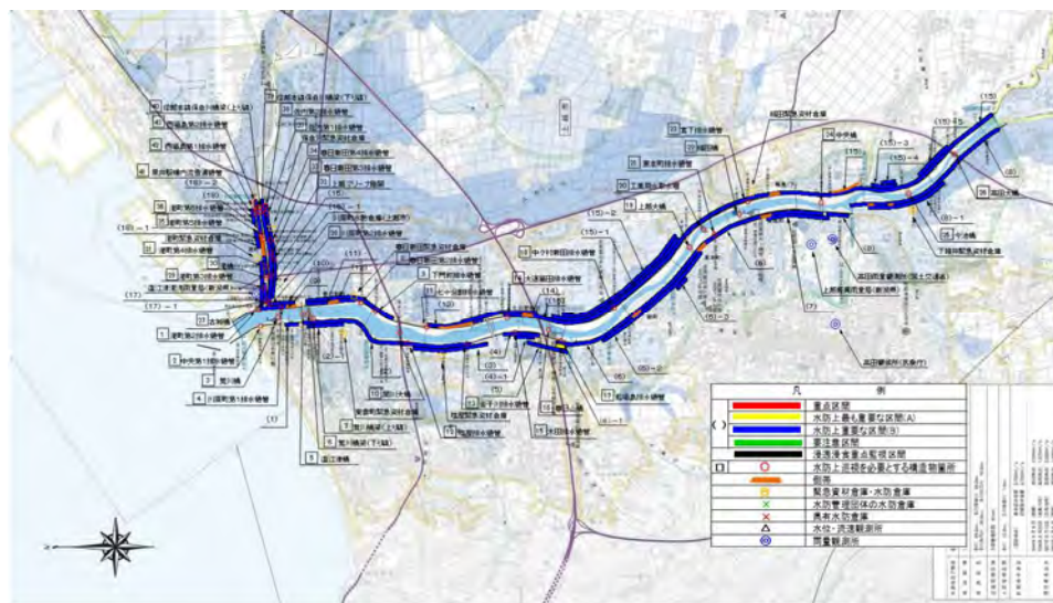
図 3-10 関川重要水防箇所（令和 5 年度（2023 年度））
