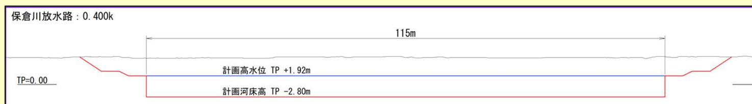
保倉川放水路の主要な地点の計画横断形状(河口付近)
