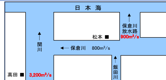
流量配分図
