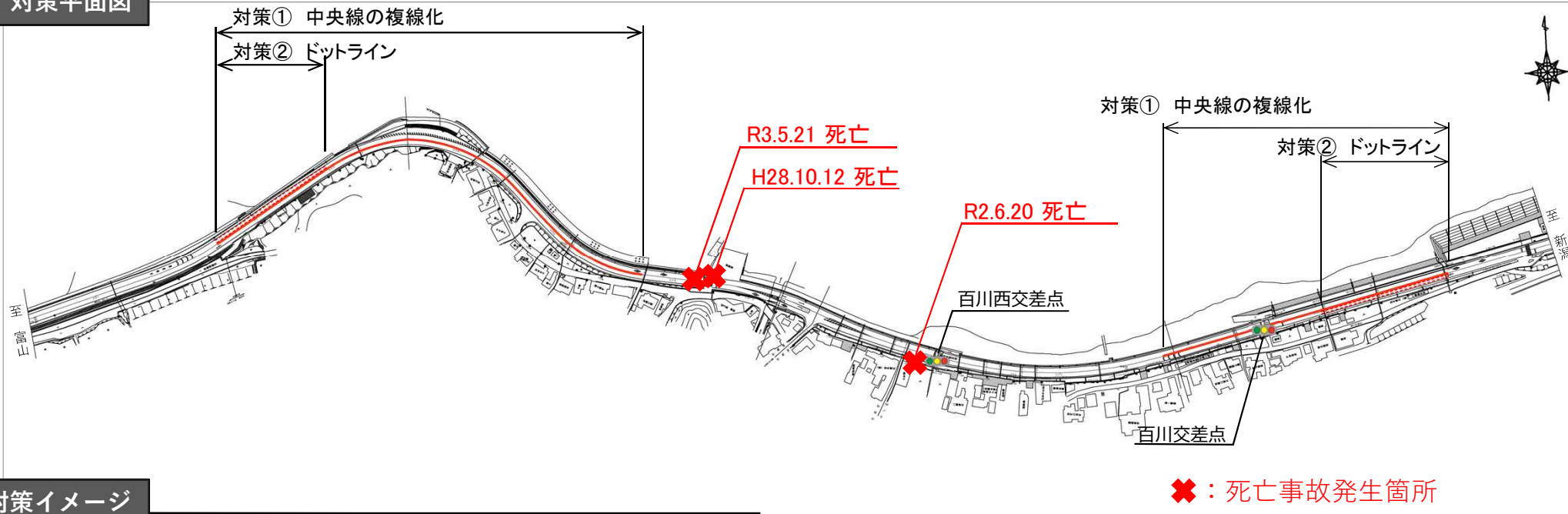
対策平面図
