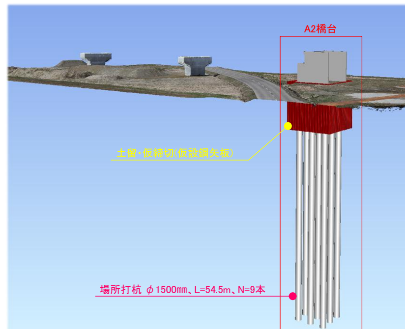
CIMモデル 完成イメージ
