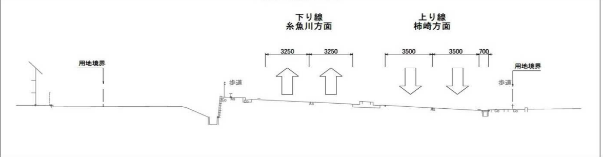
完成横断面図
