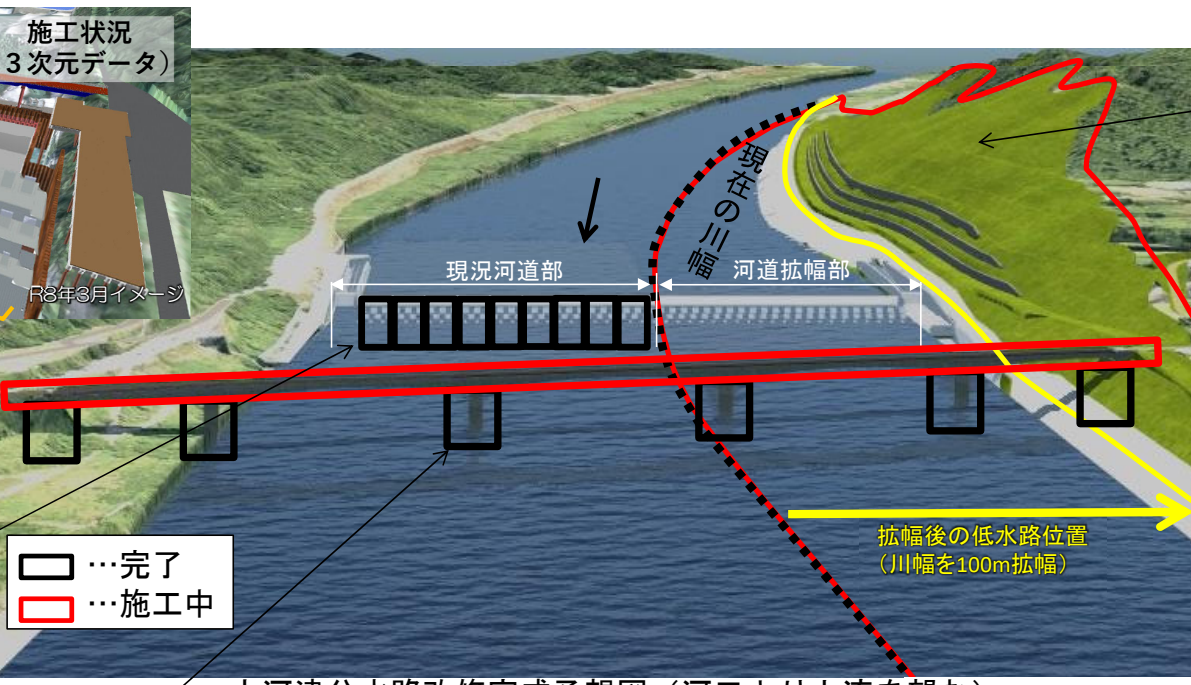
大河津分水路改修完成予想図 (河口より上流を望む)
