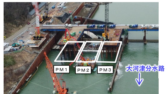
新第二床固鋼殻ケーソン (PM1～3) 据付・設置の状況 (撮影日：令和4年3月2日)
