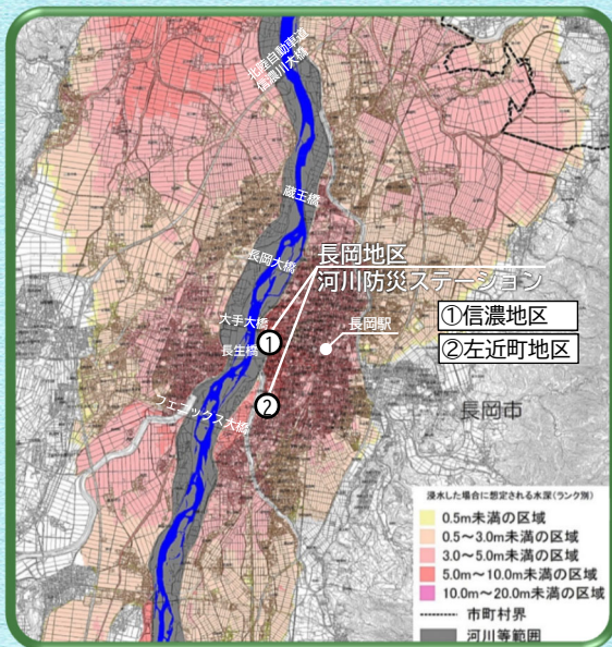
長岡地区の浸水想定区域図（想定最大規模）
