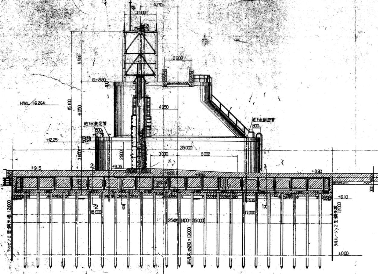
断面 S:1:100
