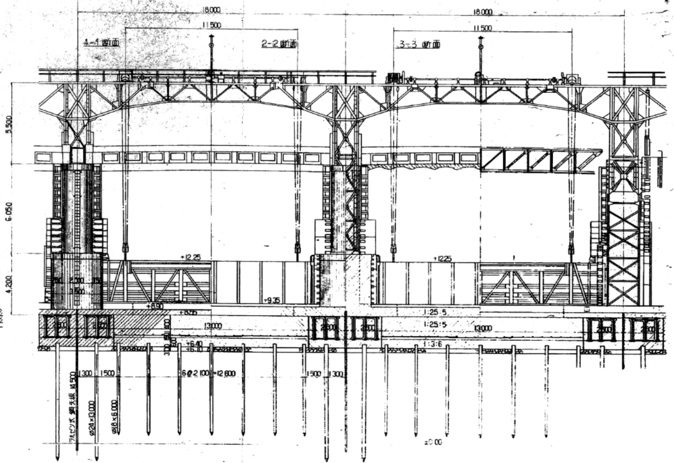
径間詳細図
