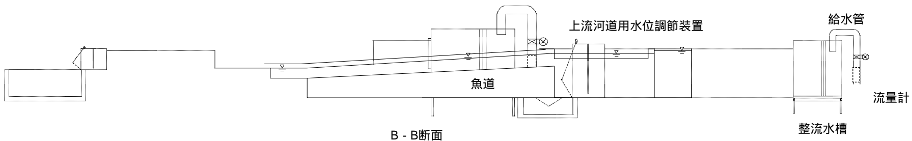
【縦断配置図】
