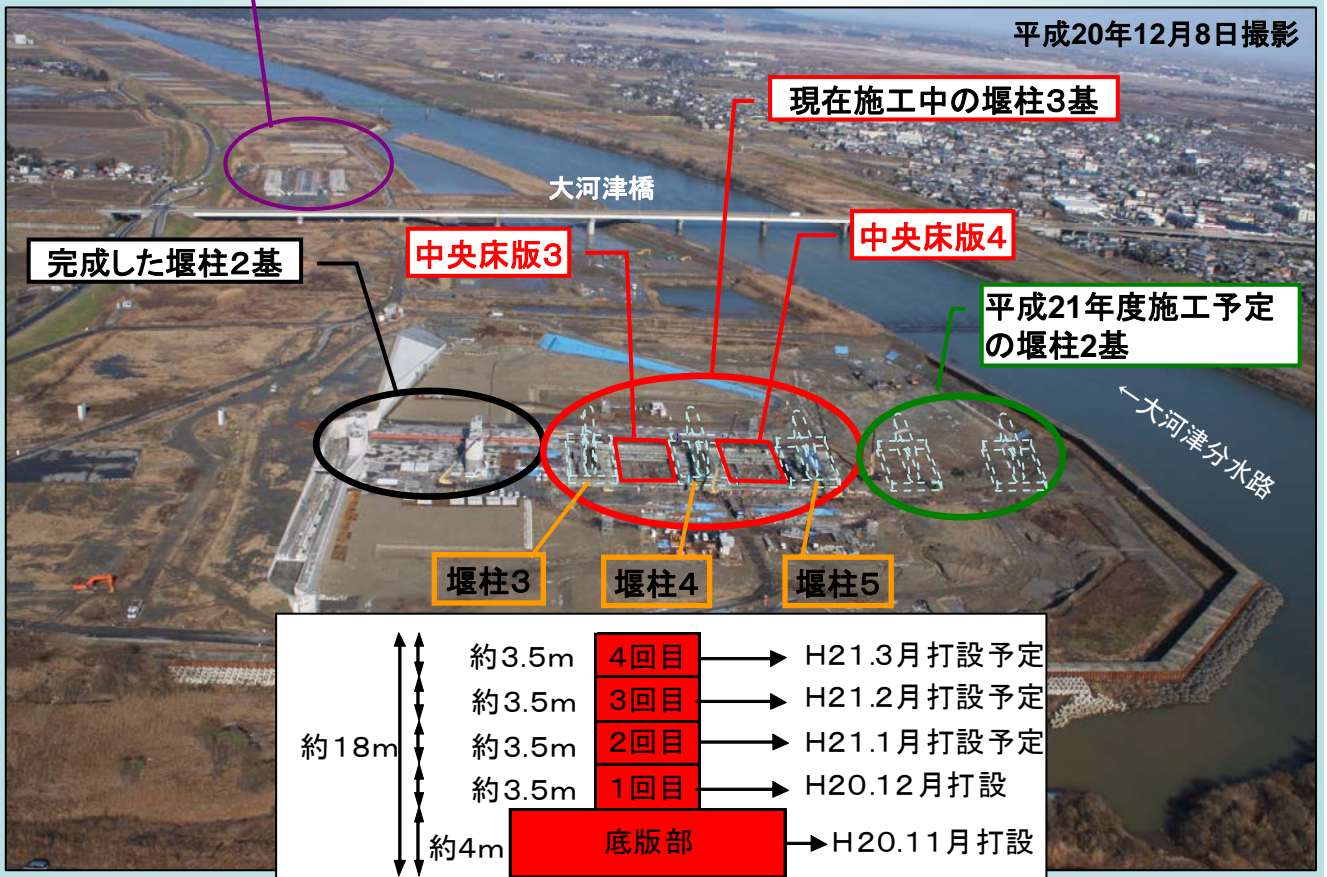
堰柱3、堰柱4、堰柱5のコンクリート打設の順序
