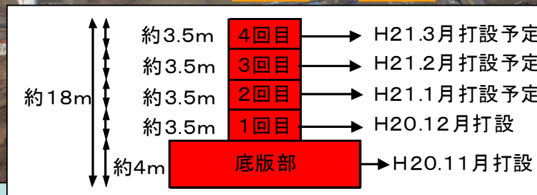
堰柱3、堰柱4、堰柱5のコンクリート打設の順序
