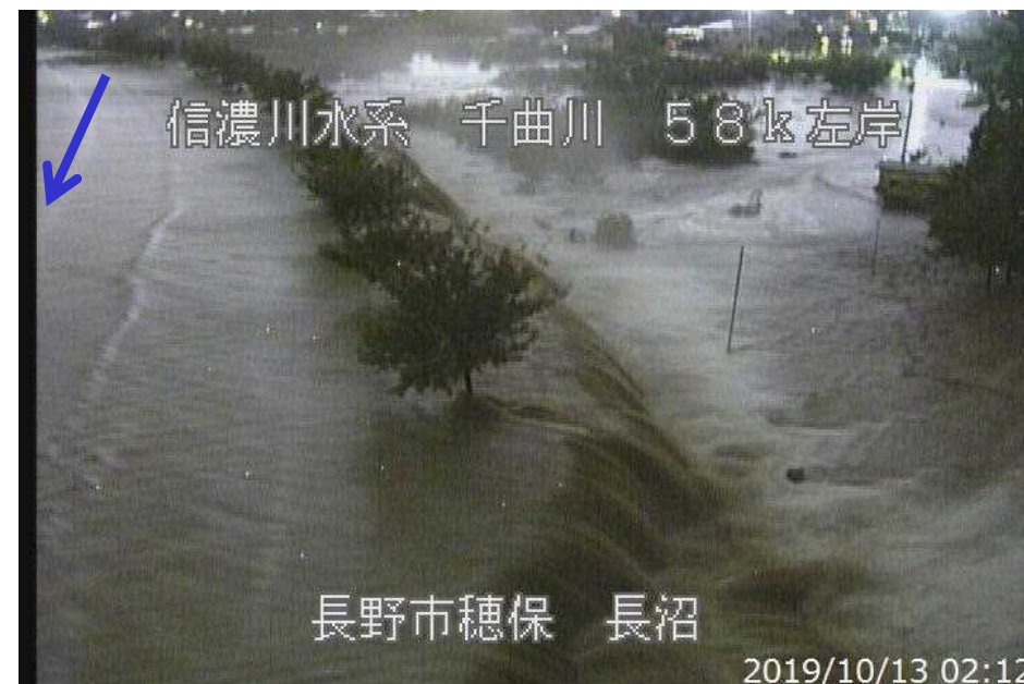
決壊箇所越水状況(10月13日2時12分)
