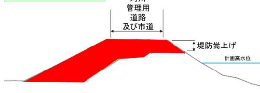
左岸:標準断面(図3-8)
