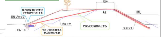
断面イメージ(図3-14)
