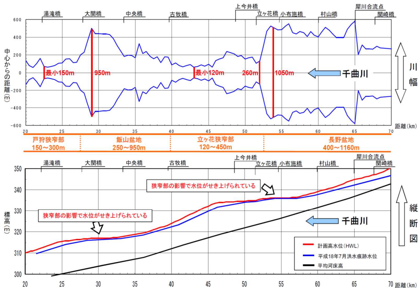
図 11 川幅と水位縦断面図
