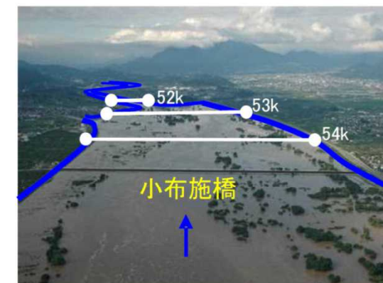
平成18年7月洪水の せき上げ状況
