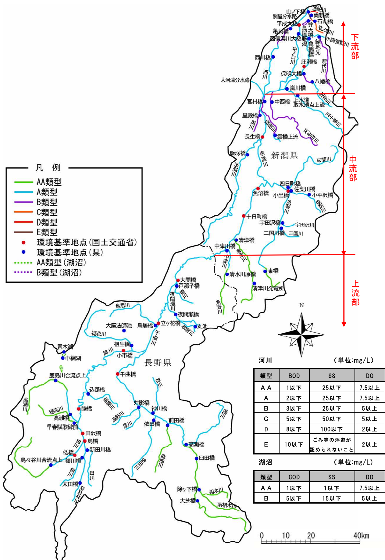
図 27 信濃川水系における河川・湖沼の水質環境基準の類型指定状況
