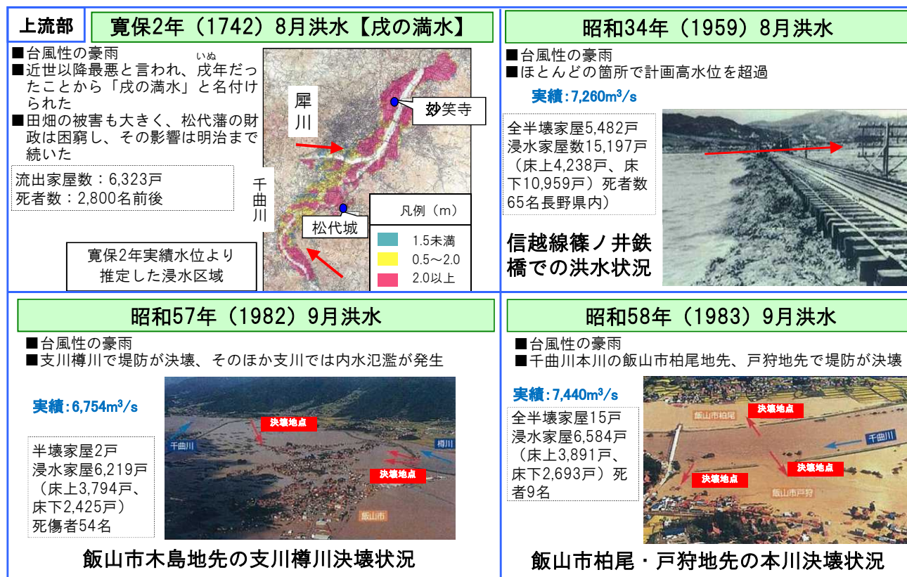
図 3 主な過去の洪水（上流部）
