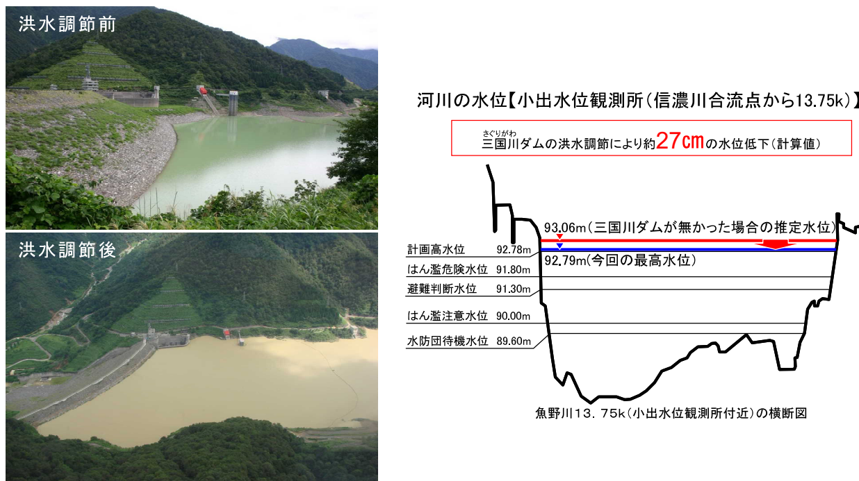
図 16 平成 23 年 7 月洪水時における三国川ダムの洪水調節の様子
