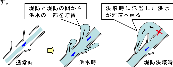
図 19 霞堤の効果
