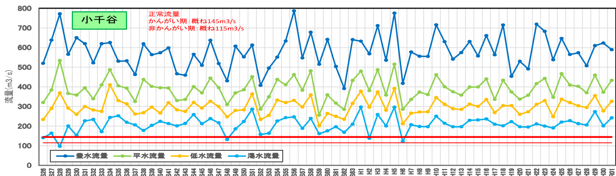
図 25 河川流況(小千谷地点)
