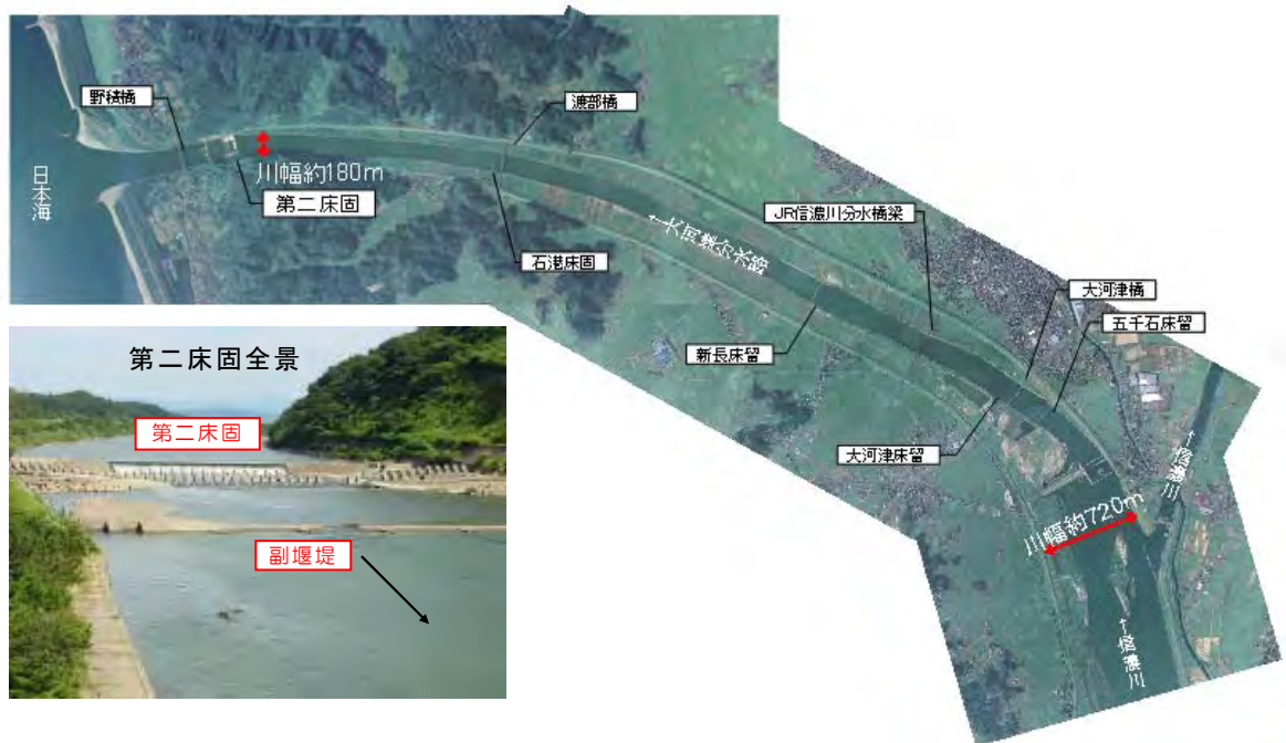
図 15 大河津分水路全体図
