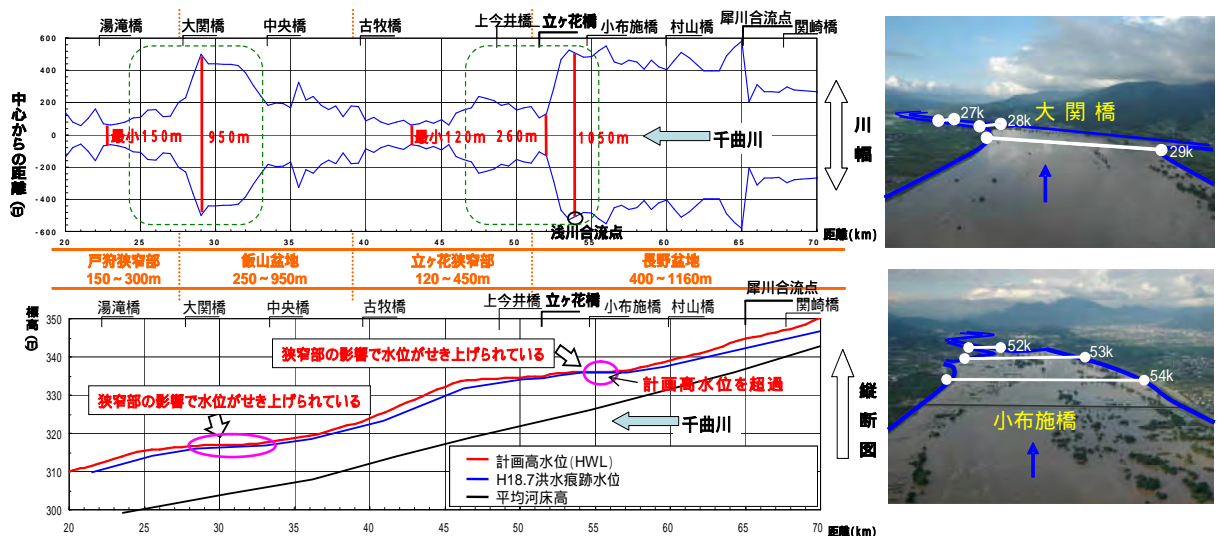
図 12 川幅と水位縦断面図
