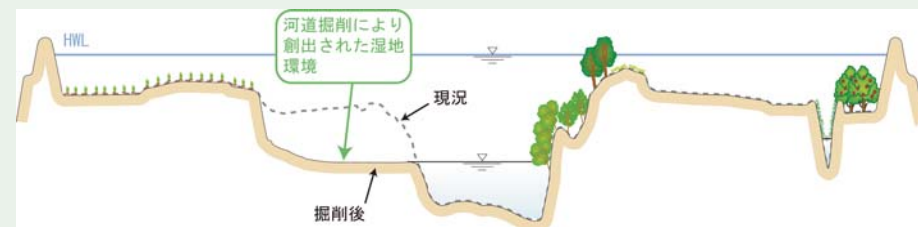
▲下流部における環境に配慮した河道横断形状
