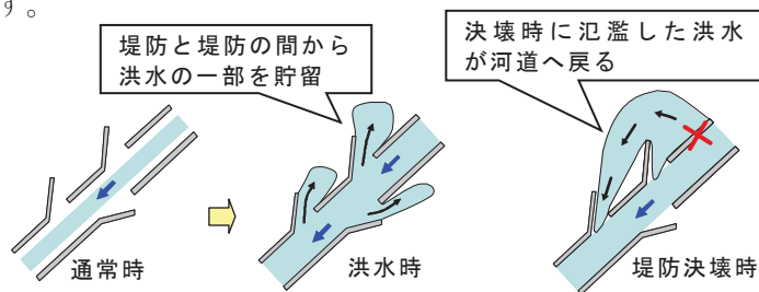
図 16 霞堤の効果
