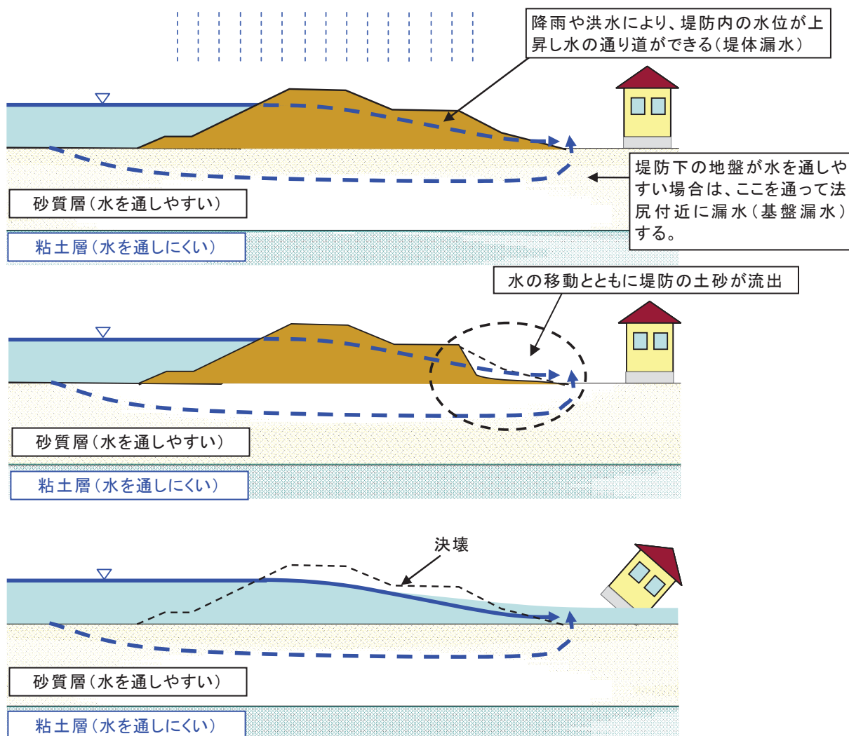
図 17 浸透による堤防の決壊メカニズム
