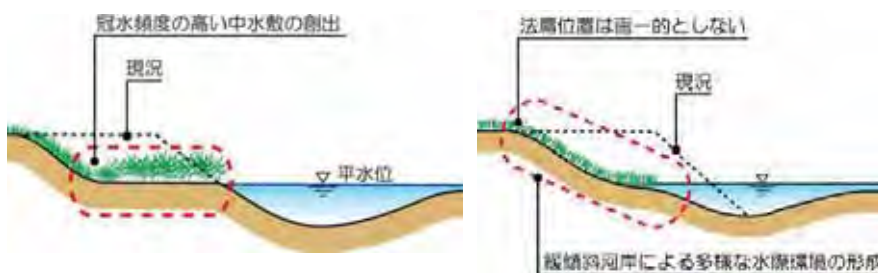
図 43 中流部における環境に配慮した河道横断形状イメージ図
