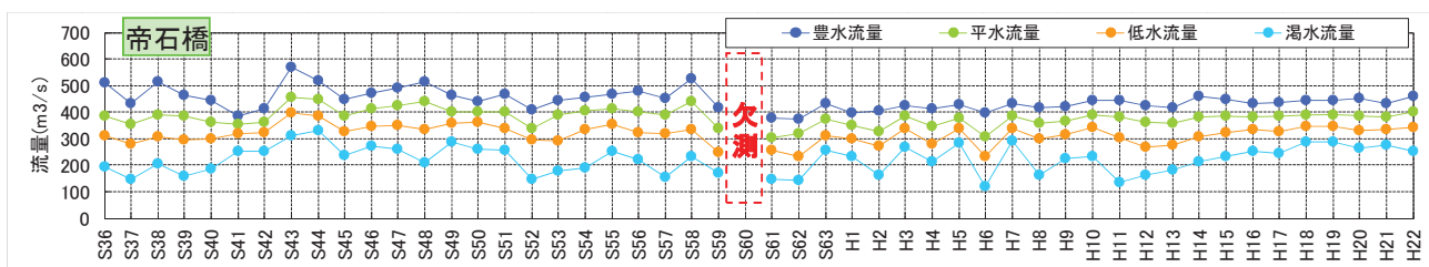
図 23 河川流況(帝石橋地点)
