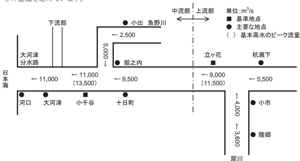
図6 河川整備基本方針における上流部・中流部計画高水流量図 (単位:m³/s)
