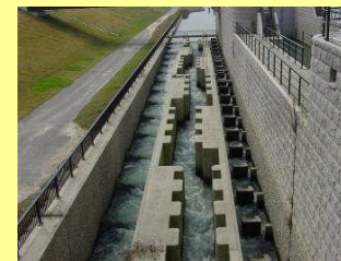
大河津洗堰魚道
