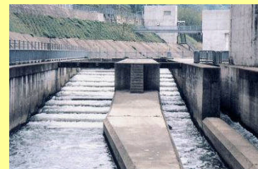
妙見堰魚道
