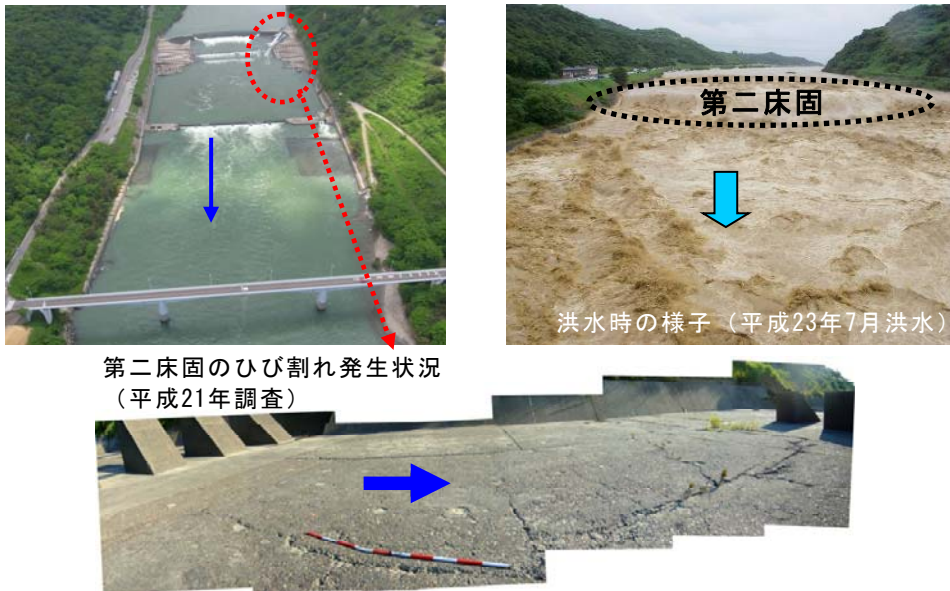
写真 17 大河津分水路 第二床固の老朽化状況
