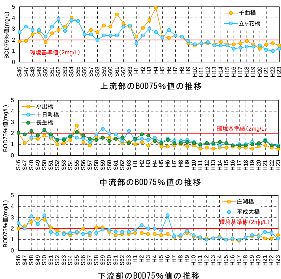
図 29 主要地点の BOD75%値の経年変化
