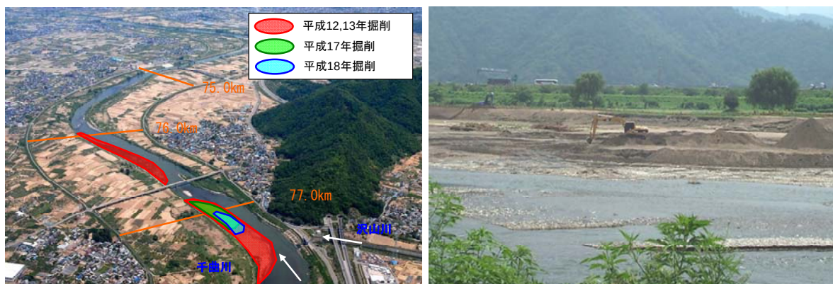
図 41 維持掘削の実施状況(千曲川沢山川合流点付近)
