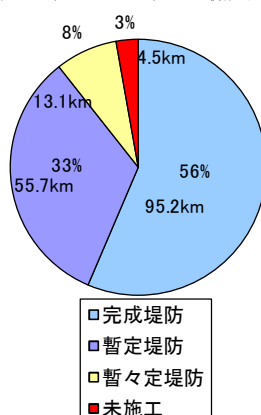
図9 中流部の堤防整備状況
