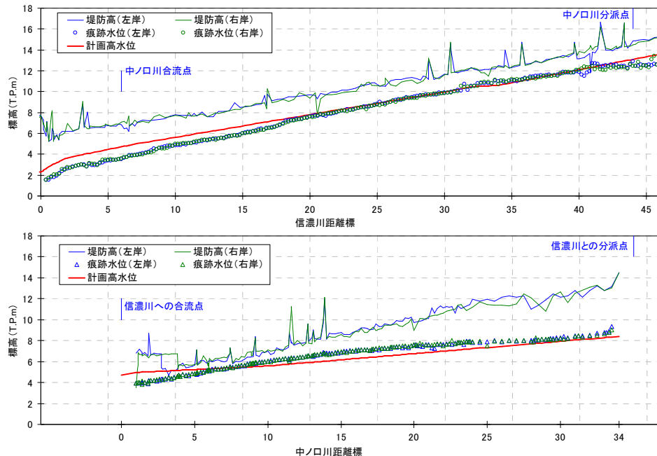
図 13 平成23年7月洪水痕跡水位縦断面図
