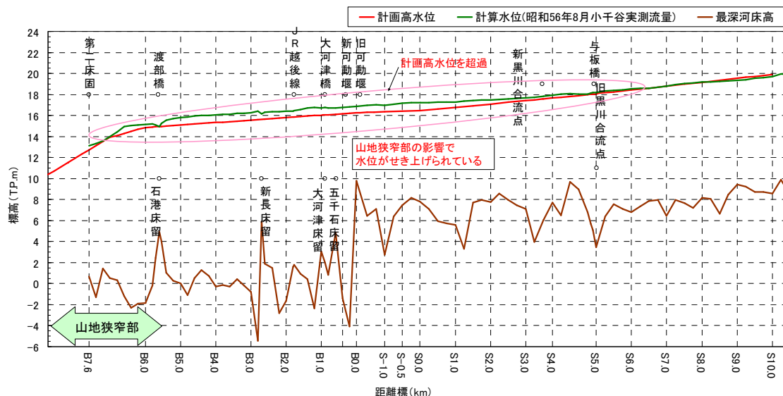
図 12 昭和56年8月洪水水位縦断面図(河口～信濃川10.0km)
