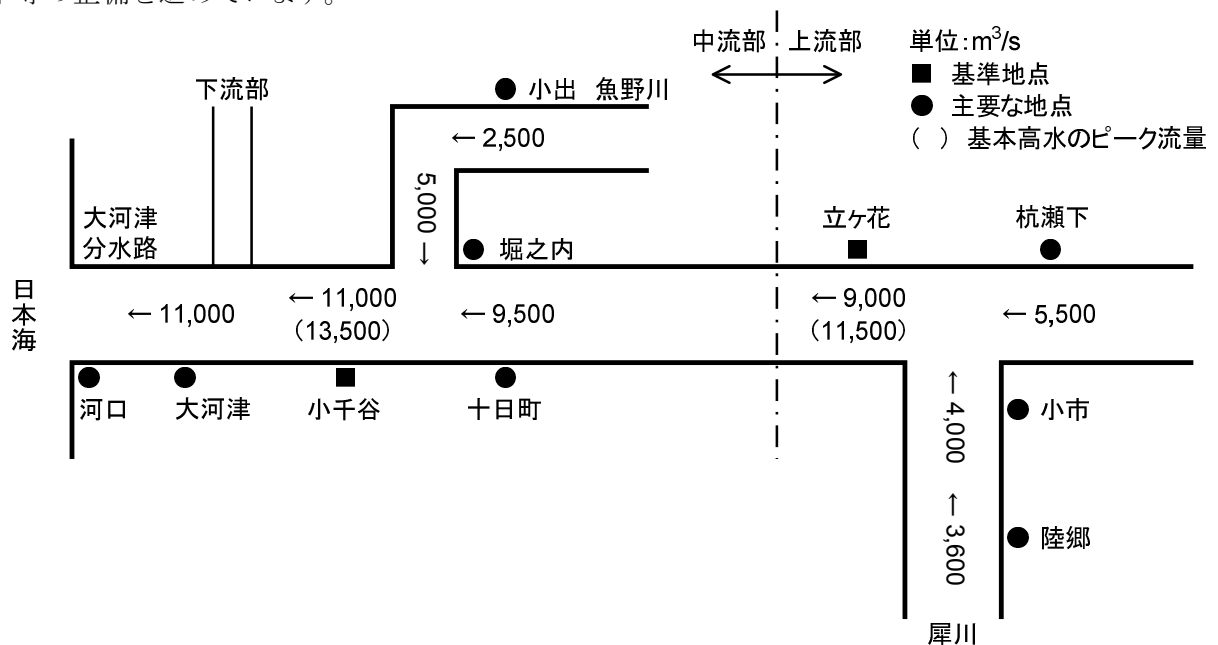
図6 河川整備基本方針における上流部・中流部計画高水流量図 (単位:m³/s)
