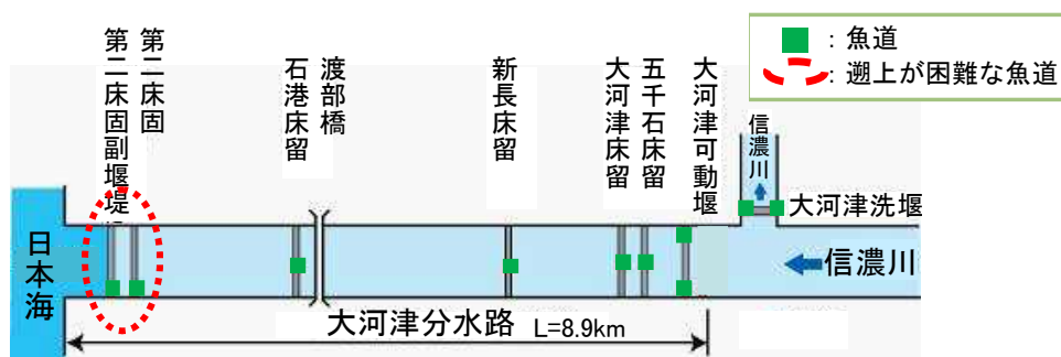
図 46 大河津分水路周辺の魚道設置状況
