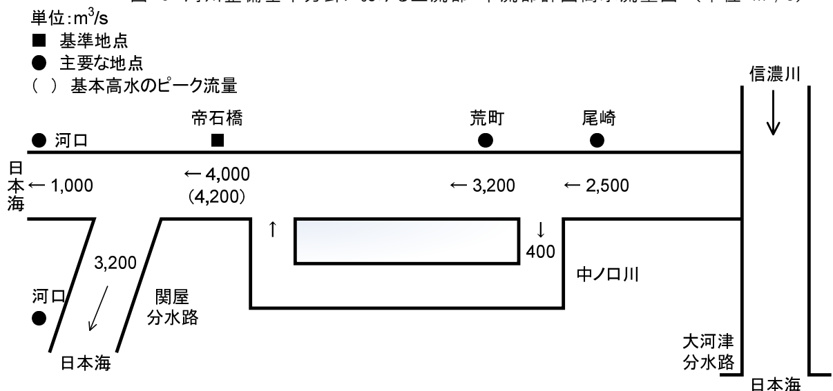
図7 河川整備基本方針における下流部計画高水流量図 (単位:m³/s)
