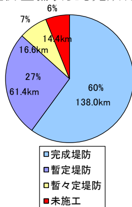
図8 上流部の堤防整備状況
