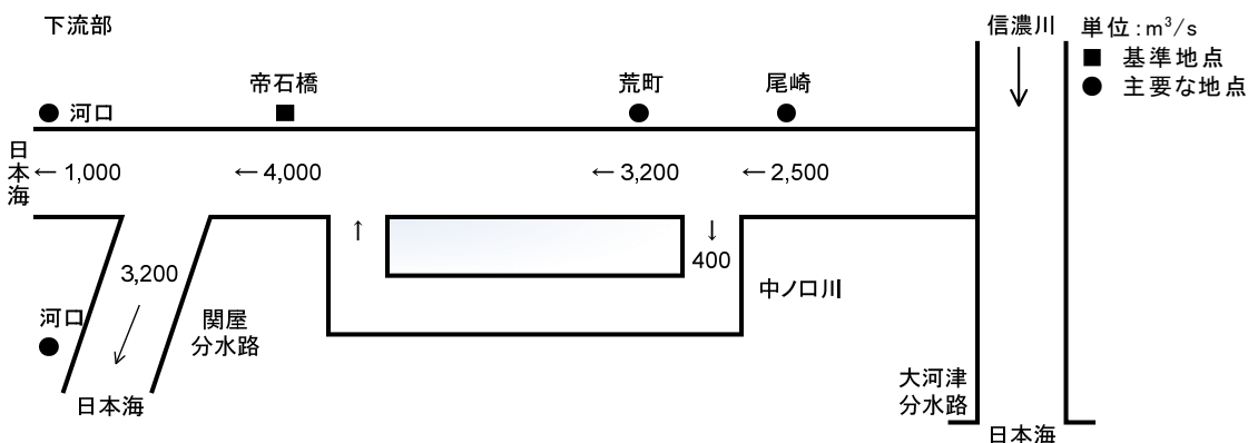
図 8 下流部計画高水流量図 (単位:m³/s)
