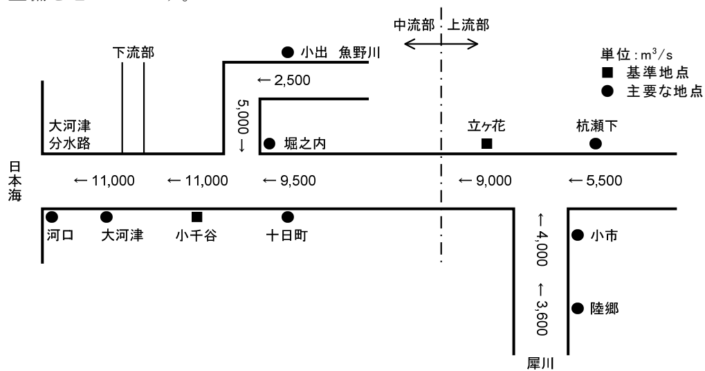
図 7 上流部・中流部計画高水流量図 (単位:m³/s)
