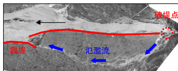
図 3-25 霞堤が効果を発揮した事例 (黒部川：昭和 44 年 8 月洪水)
