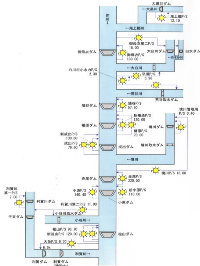
図3-33 庄川水利用模式図（上流）
