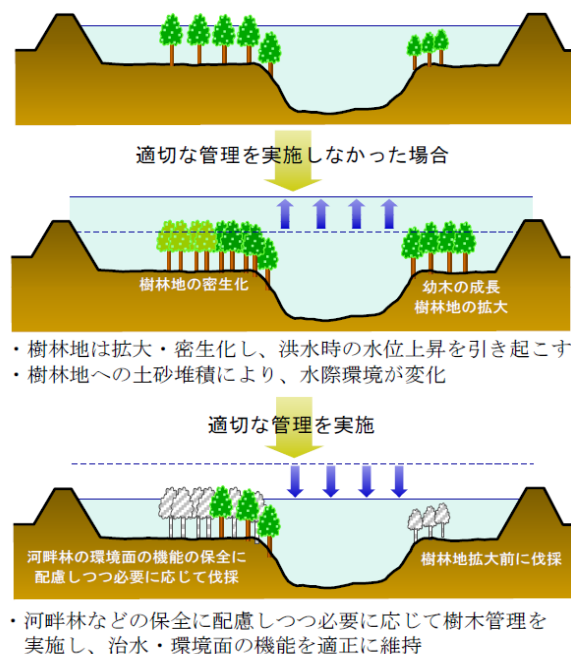
図 5-32 樹木管理イメージ（断面図）
