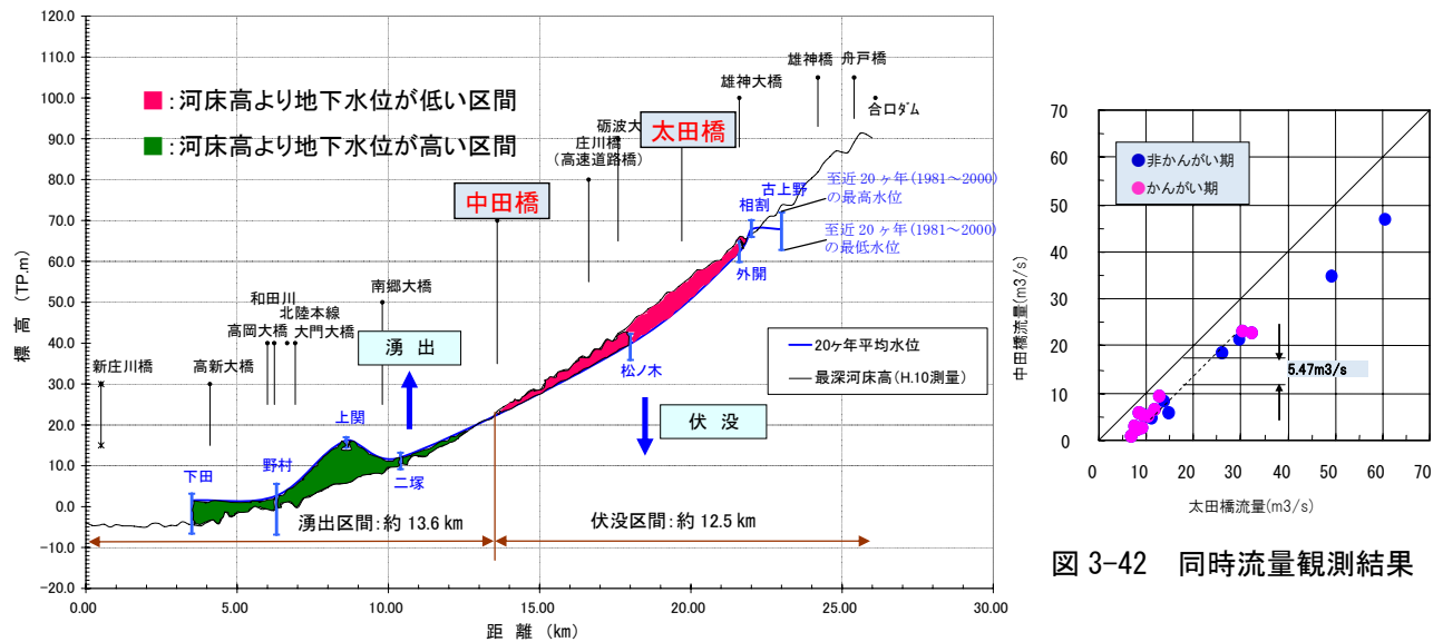
図3-41 庄川最深河床高と周辺地下水位の関係
