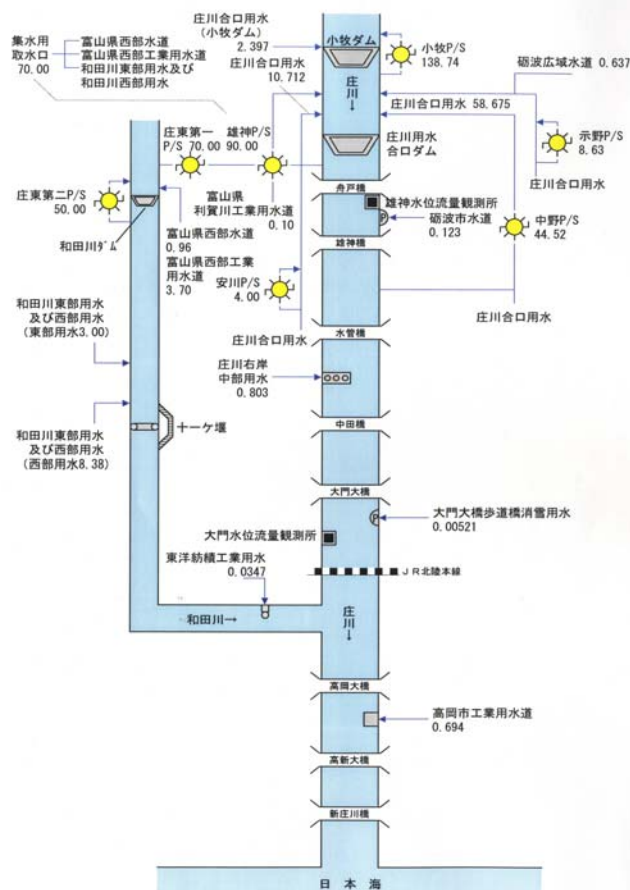
図3-34 庄川水利用模式図（下流）
