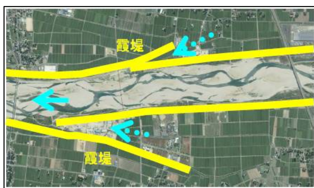
図 5-17 庄川の霞堤
