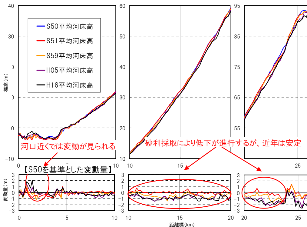
図3-19 河床高縦断の経年変化と変動量
