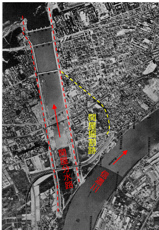
関屋分水路概成 昭和46年10月
